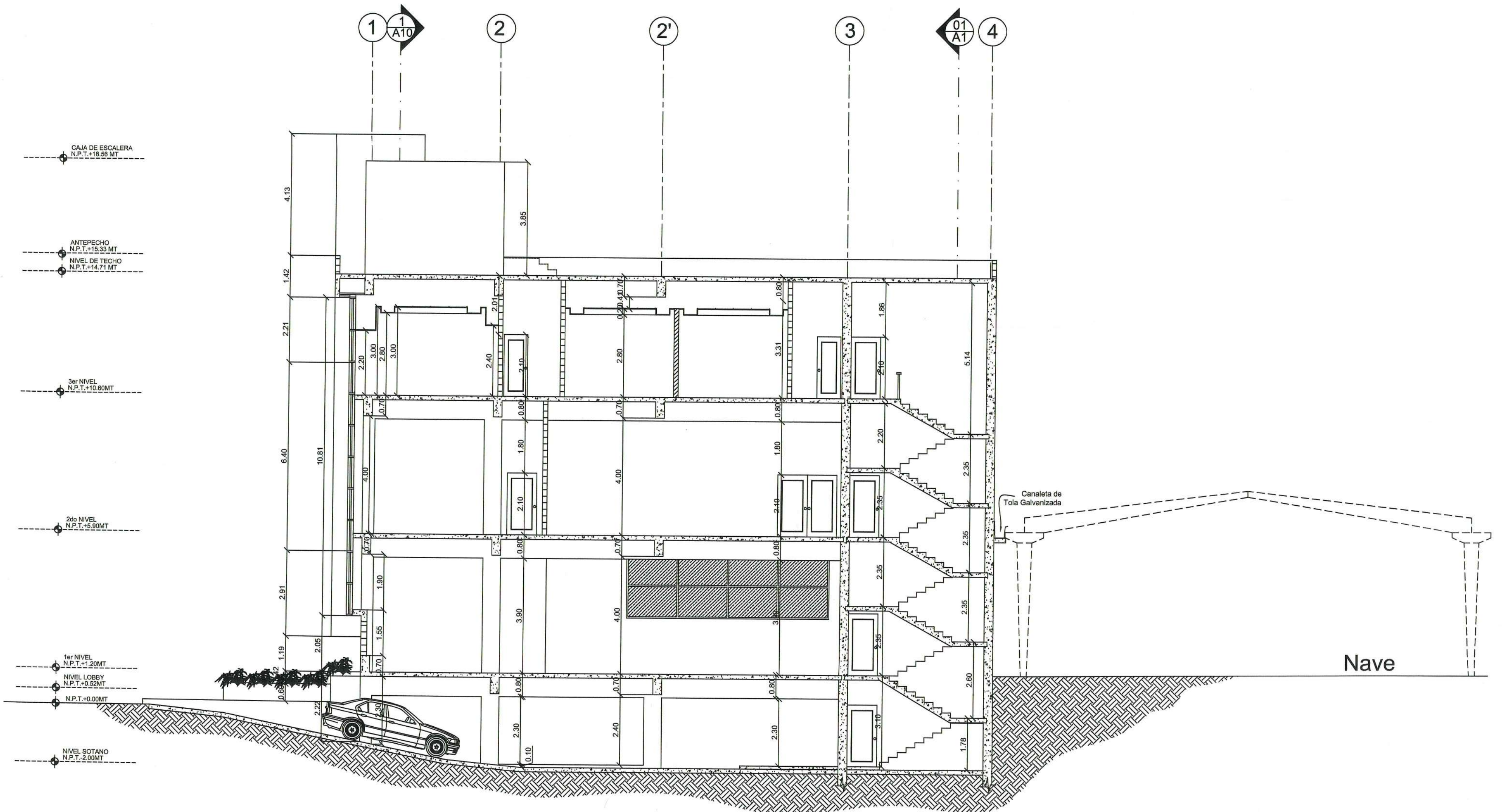
2 Seccion Transversal 2 Esc. 1:100 Oficinas y Talleres Serigraf S.A.
