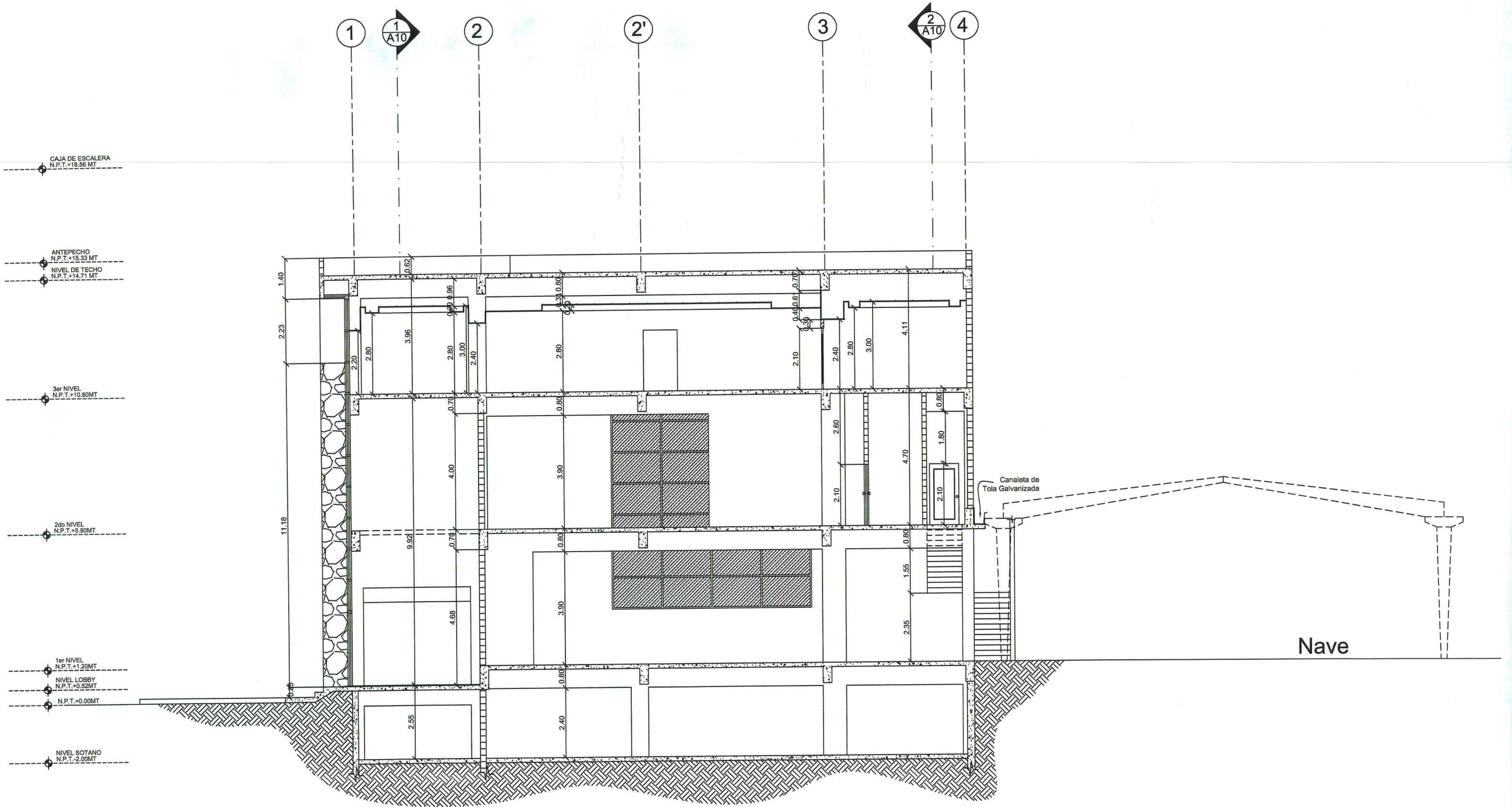
1 Seccion Transversal 3 Esc. 1:100 Oficinas y Talleres Serigraf S.A.
