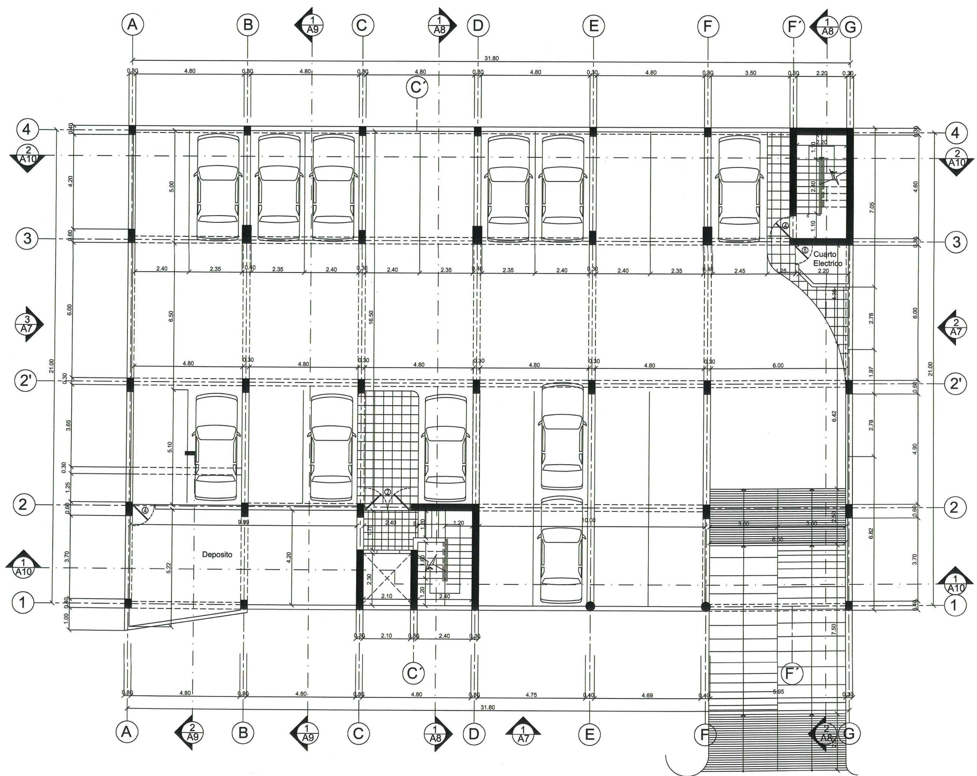
1 A1 Planta Arquitectonica Nivel de Sotano Esc. 1:100 Oficinas y Talleres Serigraf S.A.
