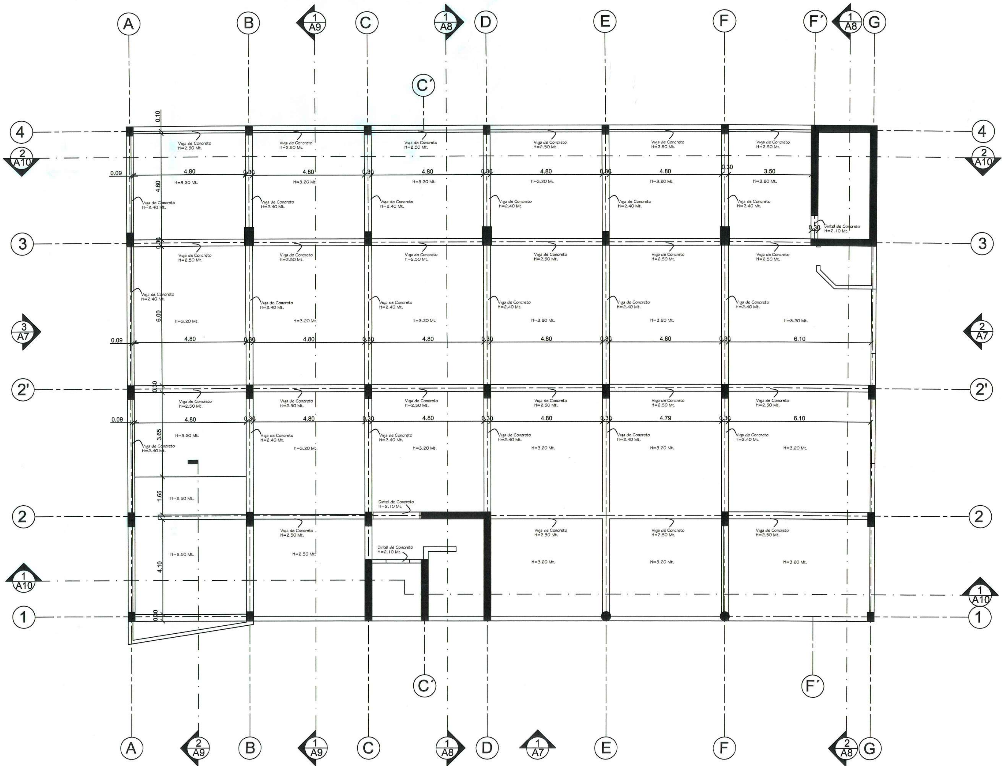
1 Plata de Techos Reflejados Sotano Esc. 1:100 Oficinas y Talleres Serigraf S.A.
