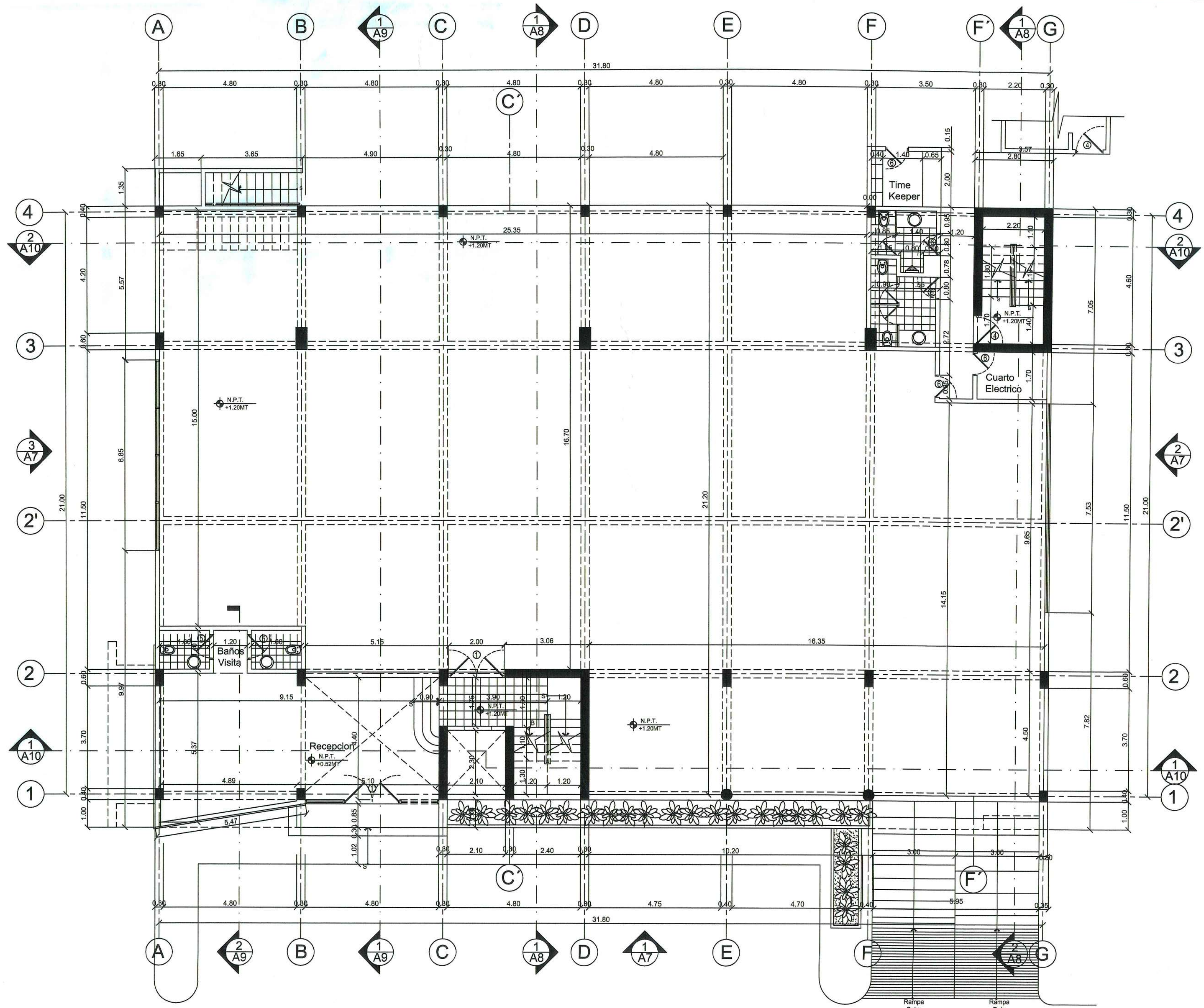
1 Planta Arquitectonica 1er Nivel Esc. 1:100 Oficinas y Talleres Serigraf S.A.
