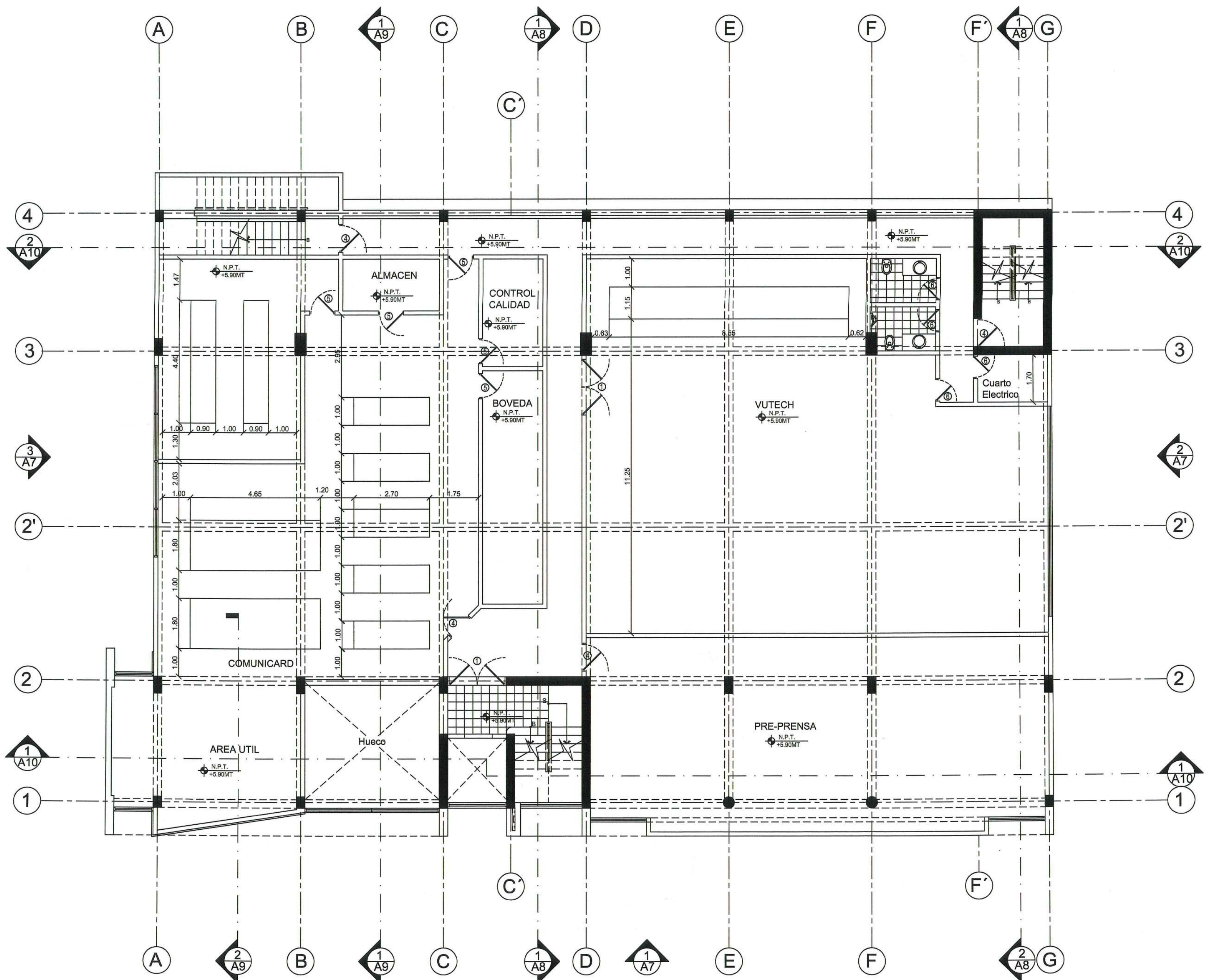
2 Planta Amueblada 2do Nivel Esc. 1:100 Oficinas y Talleres Serigraf S.A.
