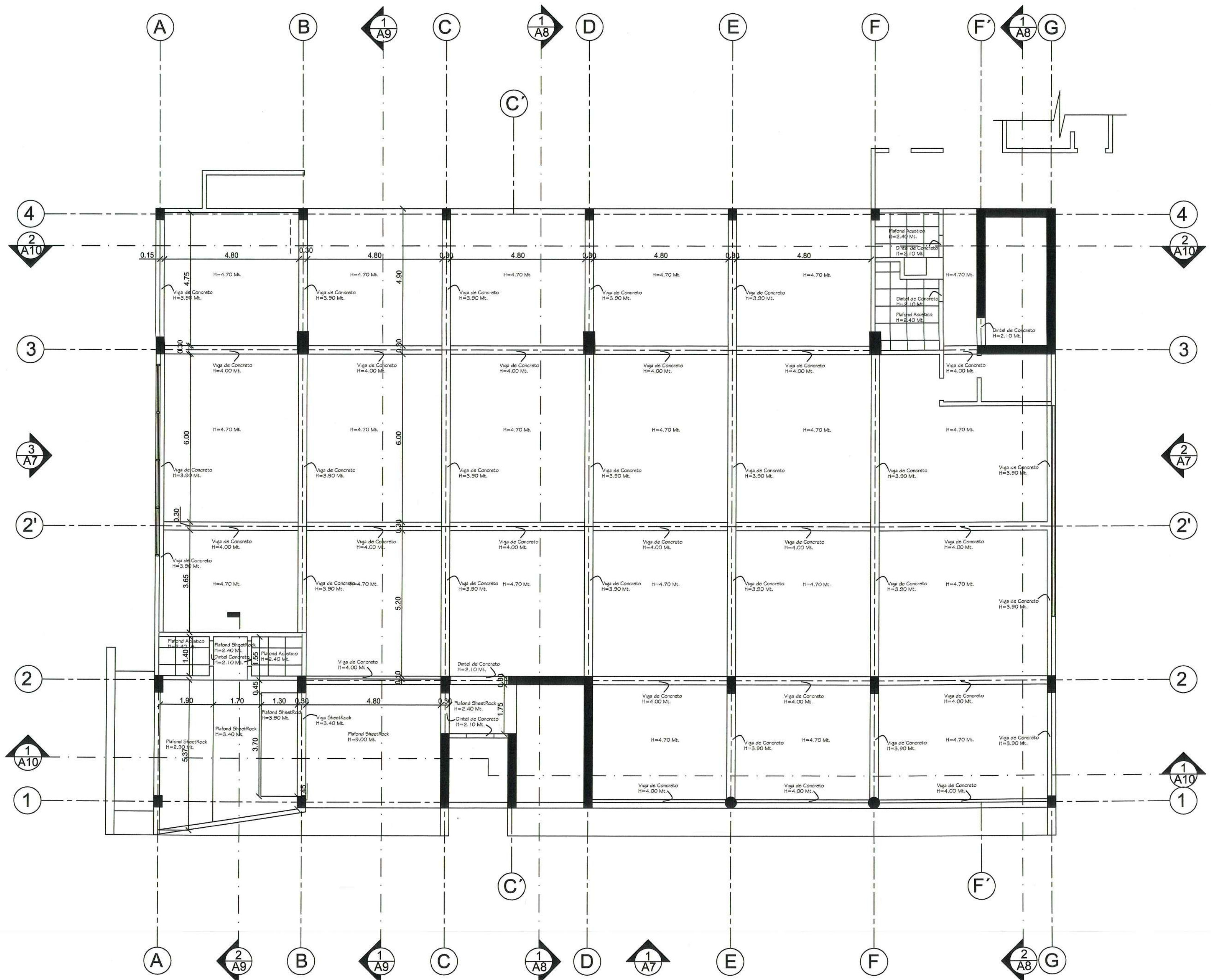
2 Planta de Techos Reflejados 1er Nivel Esc. 1:100 Oficinas y Talleres Serigraf S.A.
