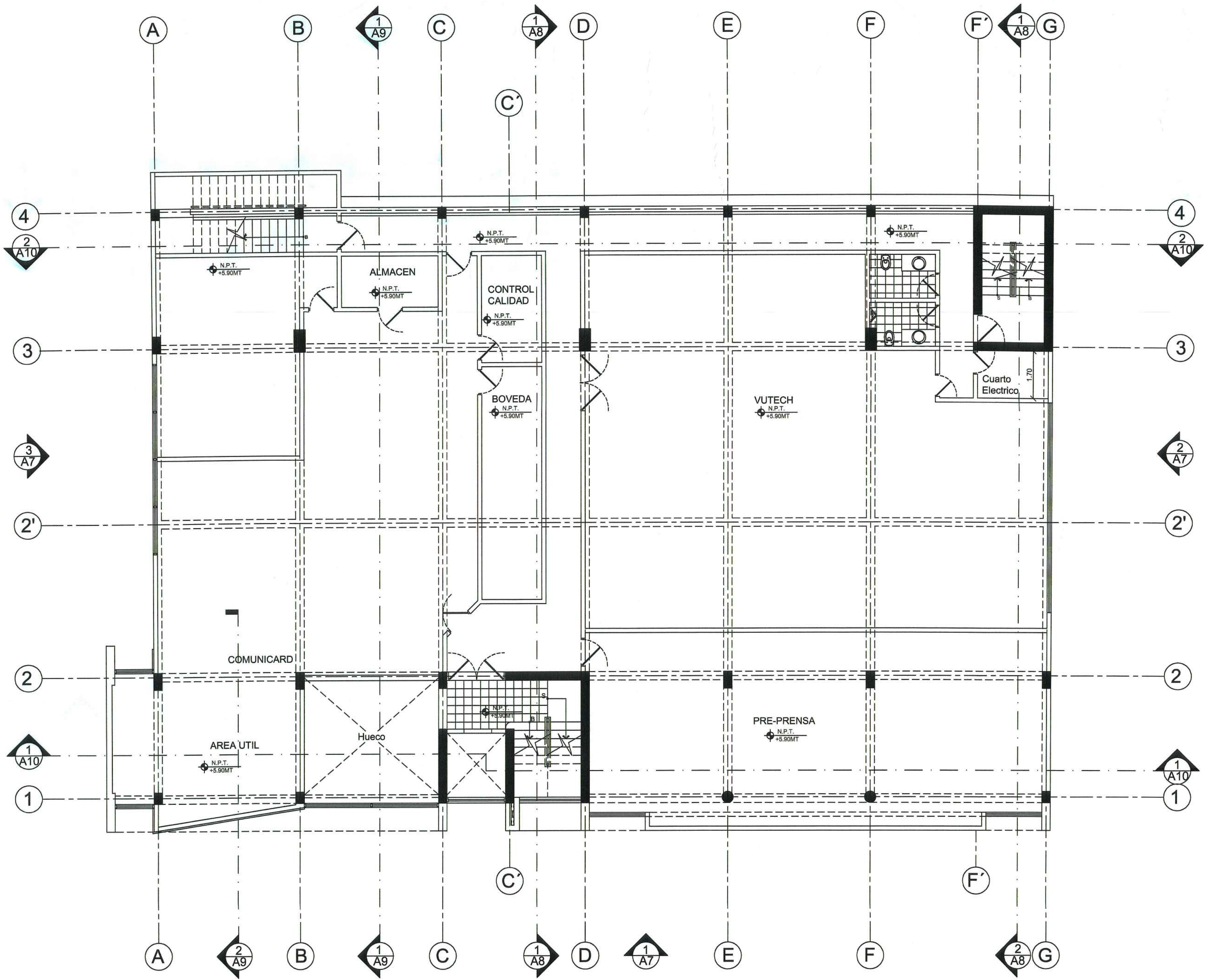
1 Planta Arquitectonica 2do Nivel Esc. 1:100 Oficinas y Talleres Serigraf S.A.
