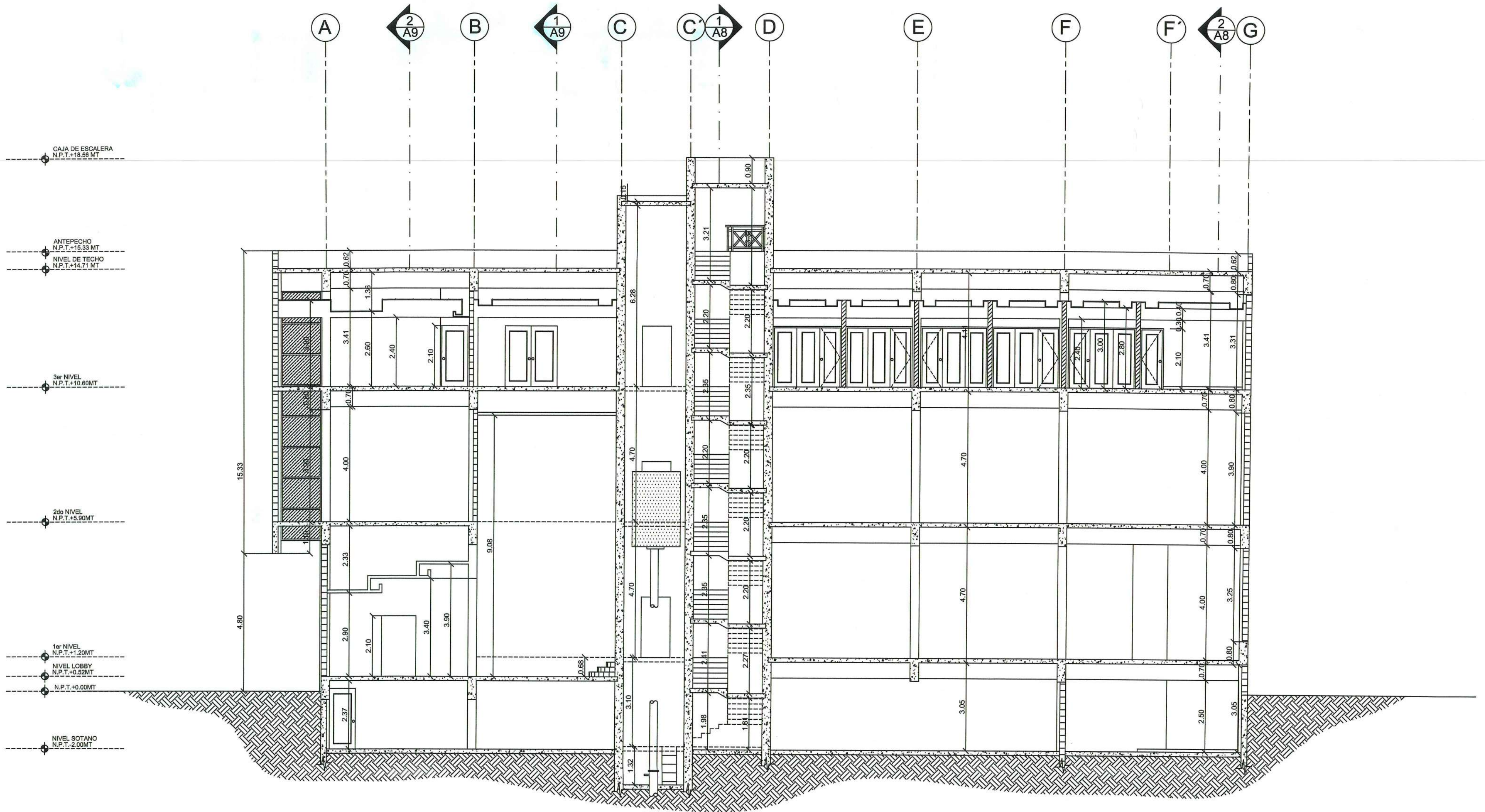
1 Seccion Longitudinal 1 Esc. 1:100 Oficinas y Talleres Serigraf S.A.
