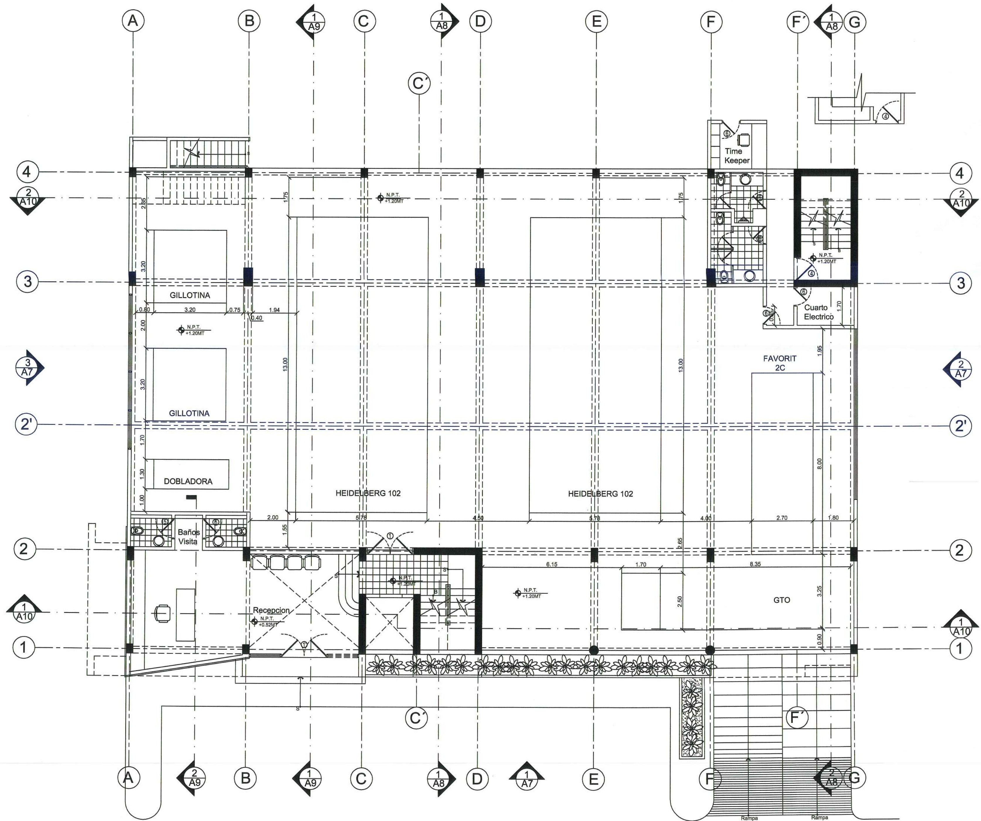
2 Planta Arquitectonica 2do Nivel Esc. 1:100 Oficinas y Talleres Serigraf S.A.
