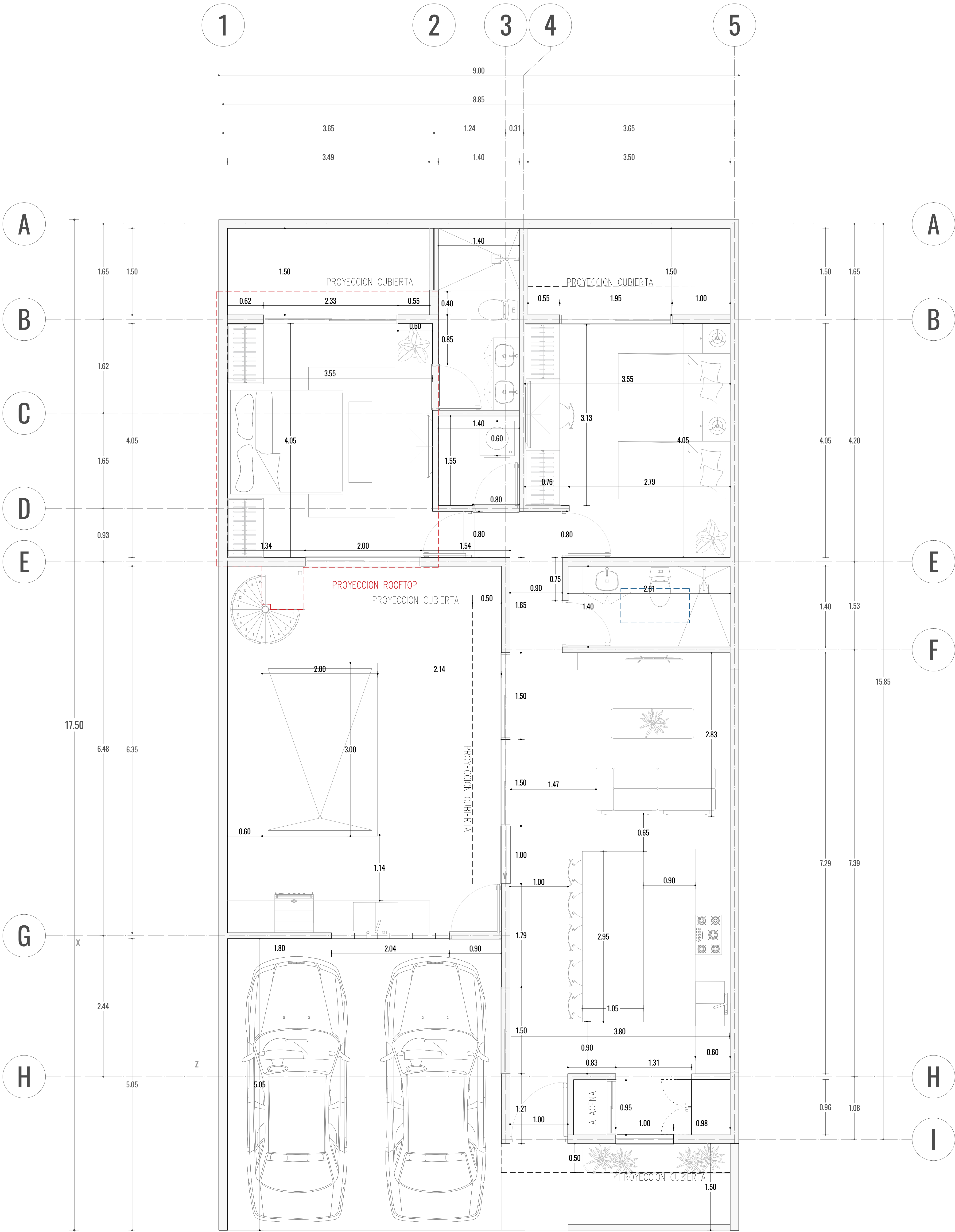
A PLANTA BAJA
