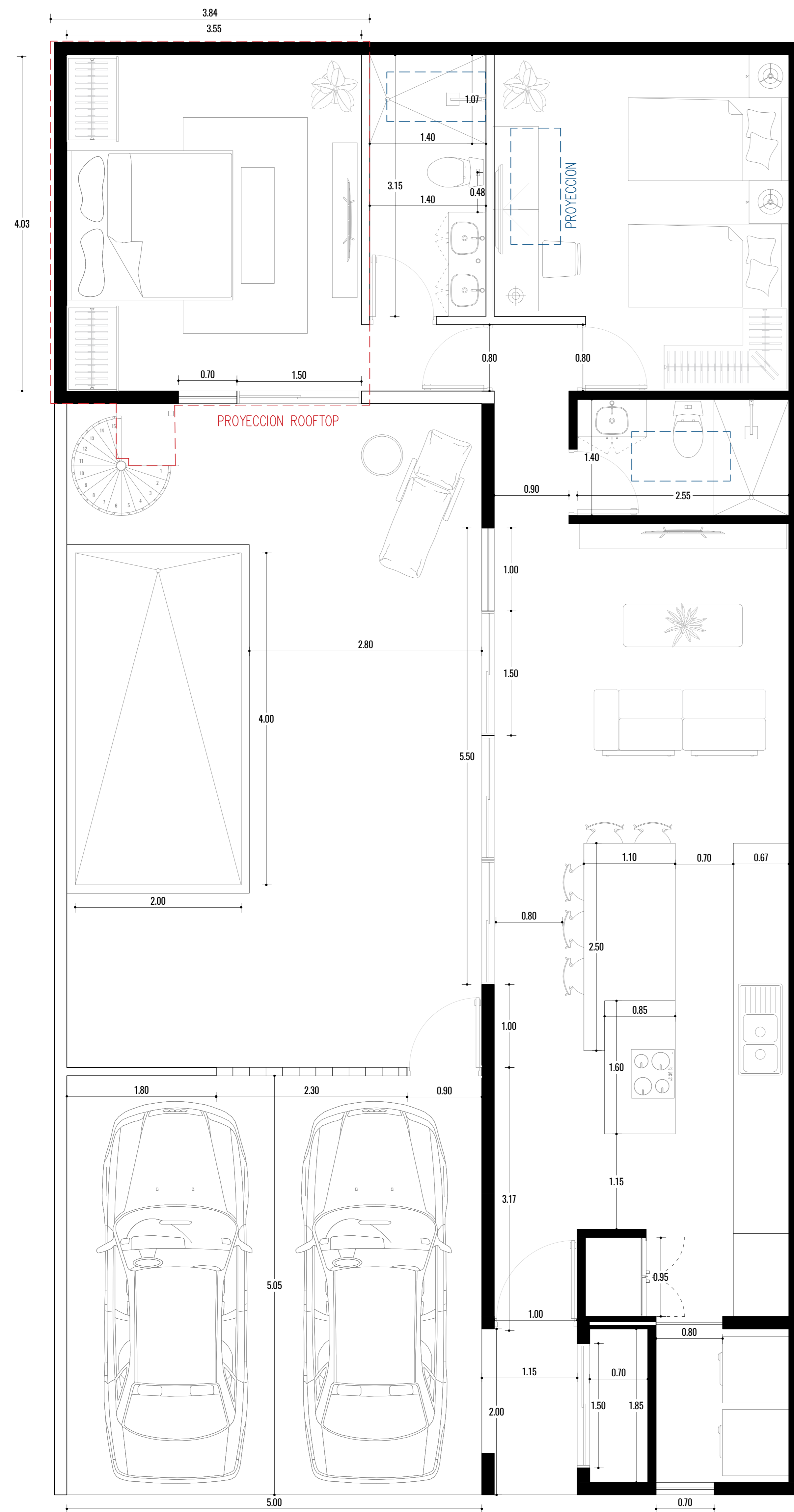
A PLANTA ARQUITECTONICA 1/30
