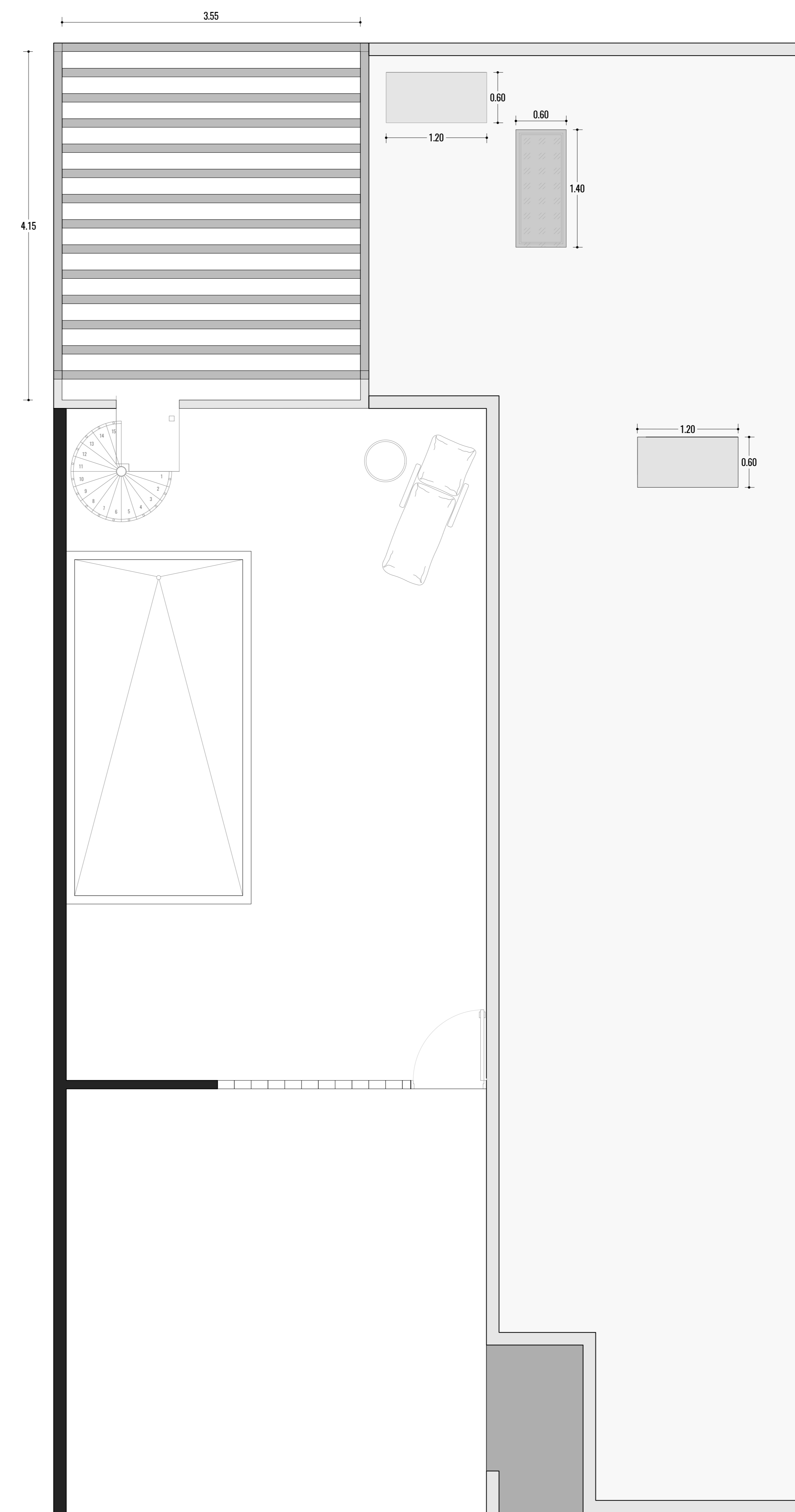
B PLANTA DE CUBIERTA 1/30
