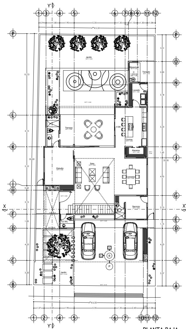
PLANTA BAJA 239.00m 2
