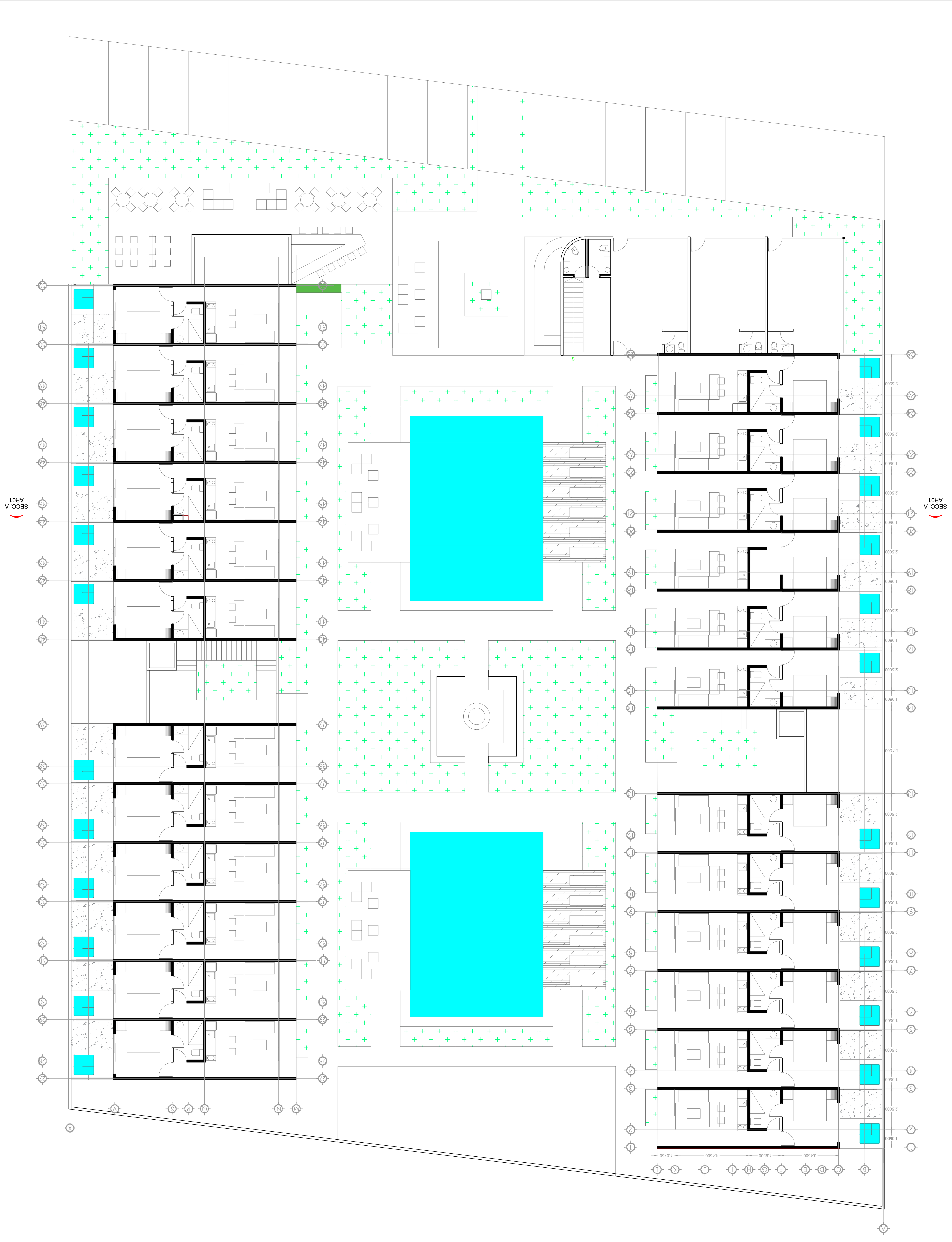
PLANTA BAJA
