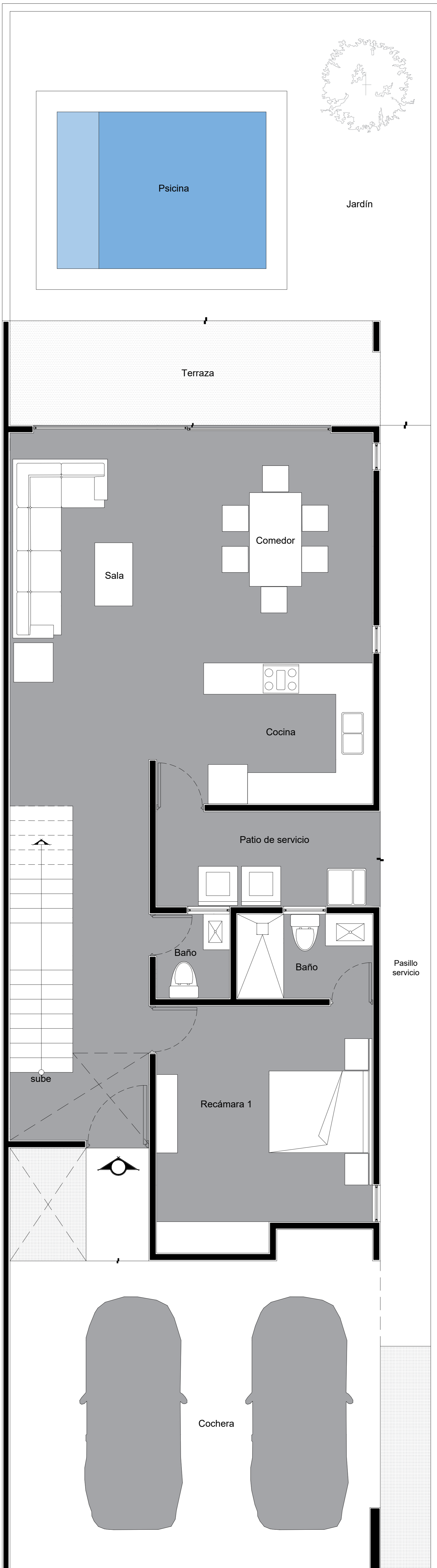
PLANTA BAJA
