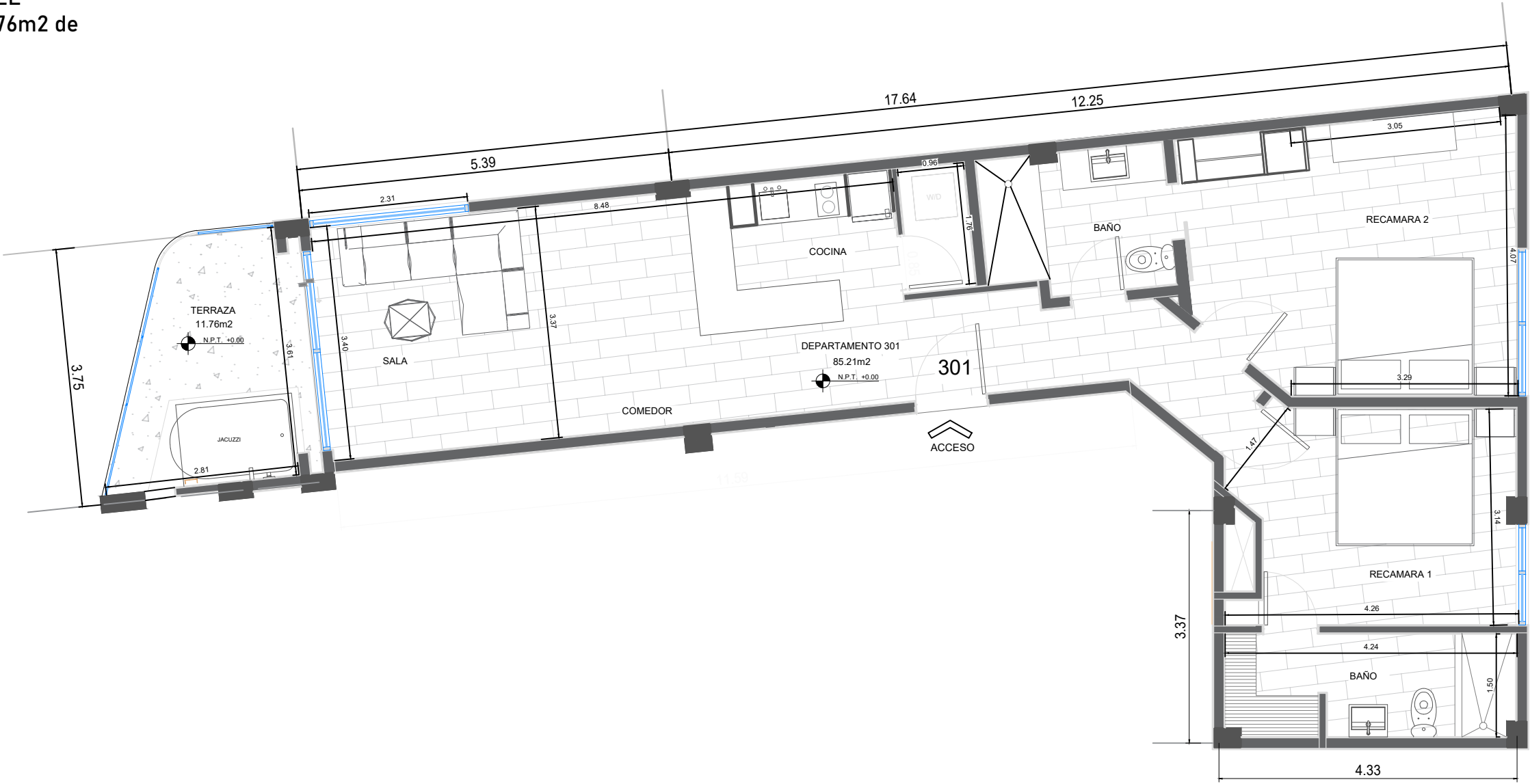
1 DEPARTAMENTO 301 ESC. 1:75
