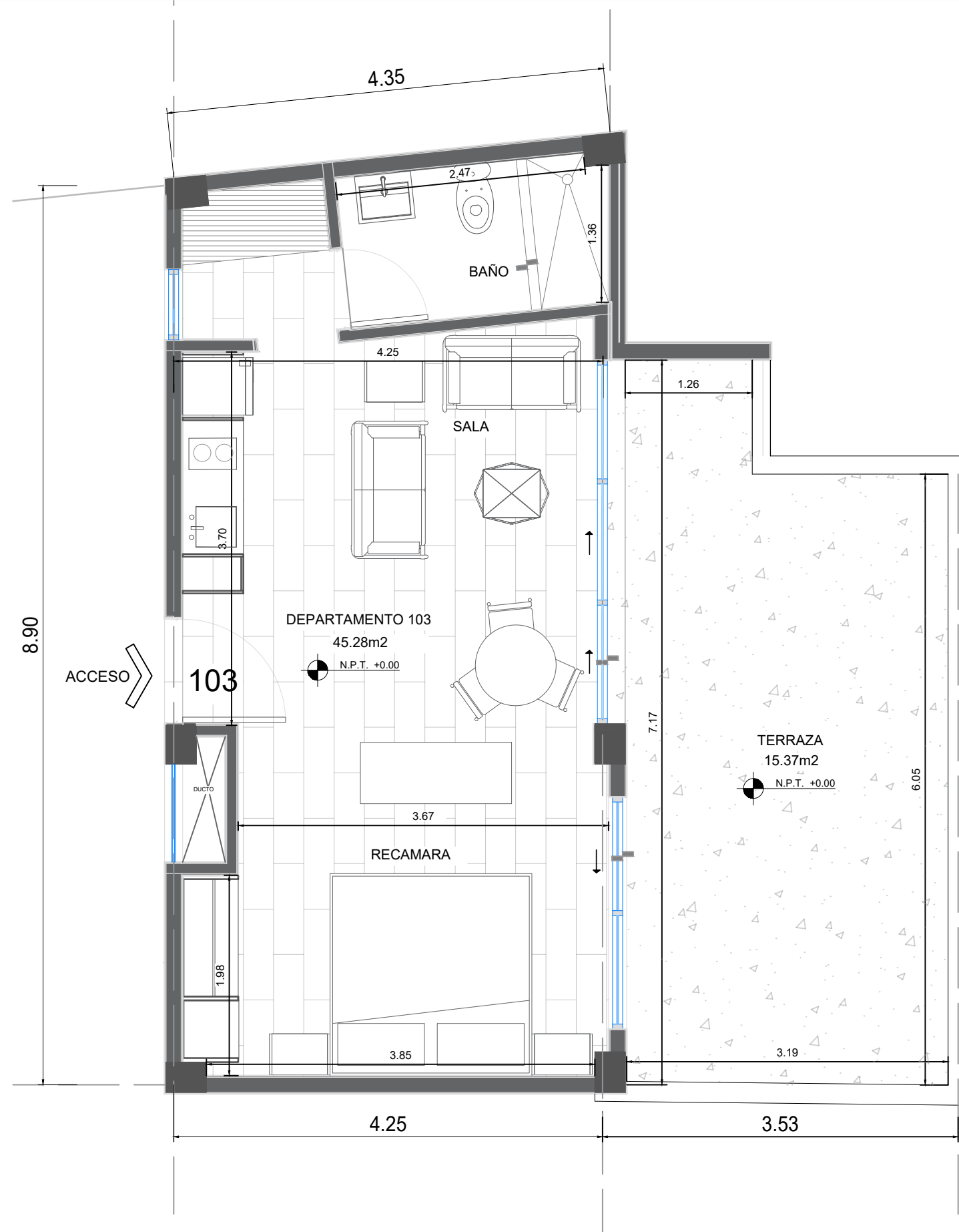
1 DEPARTAMENTO 103 ESC. 1:50
