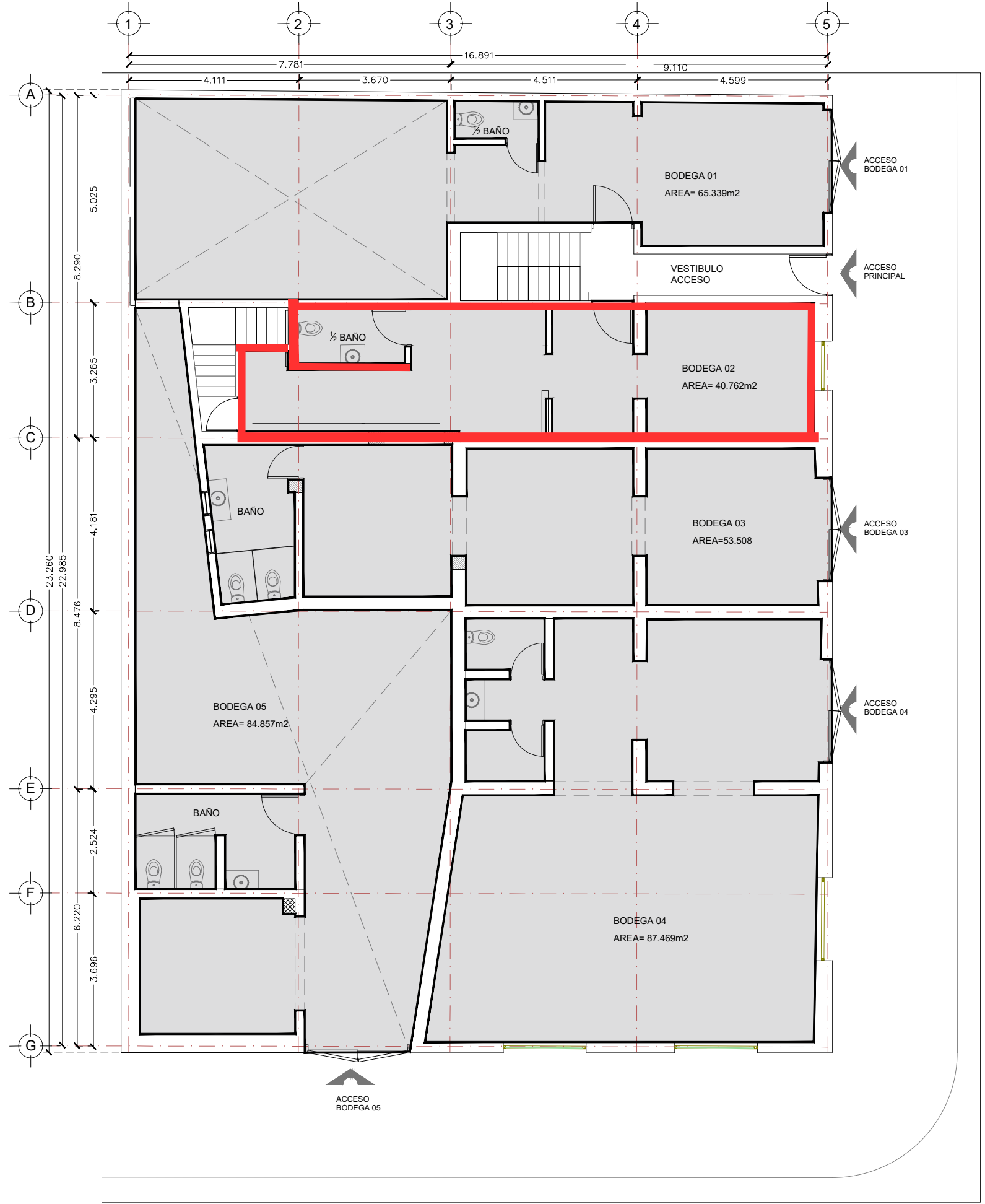
01 PLANTA BAJA ACTUALIZACIÓN DE PROYECTO 1:75
