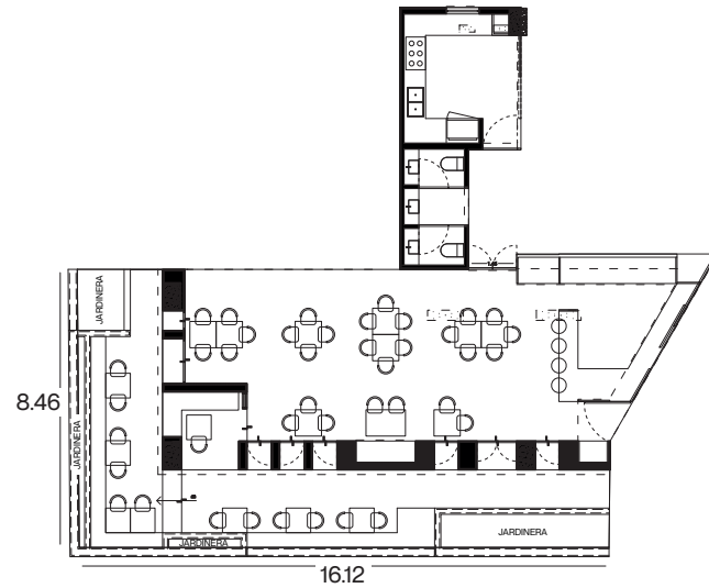
PLANTA DE LOCAL
