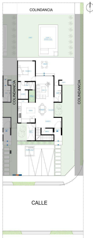
PLANTA BAJA
