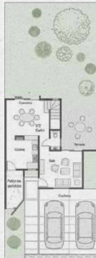
Planta baja
