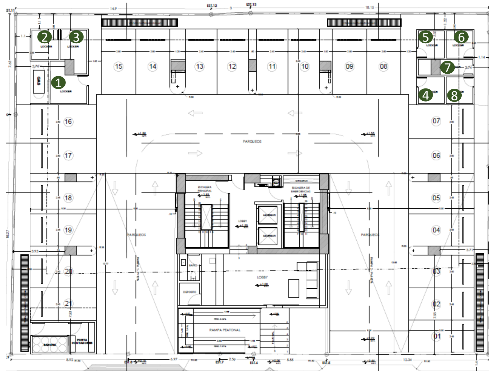
PLANTA ARQ. 1ER NIVEL
