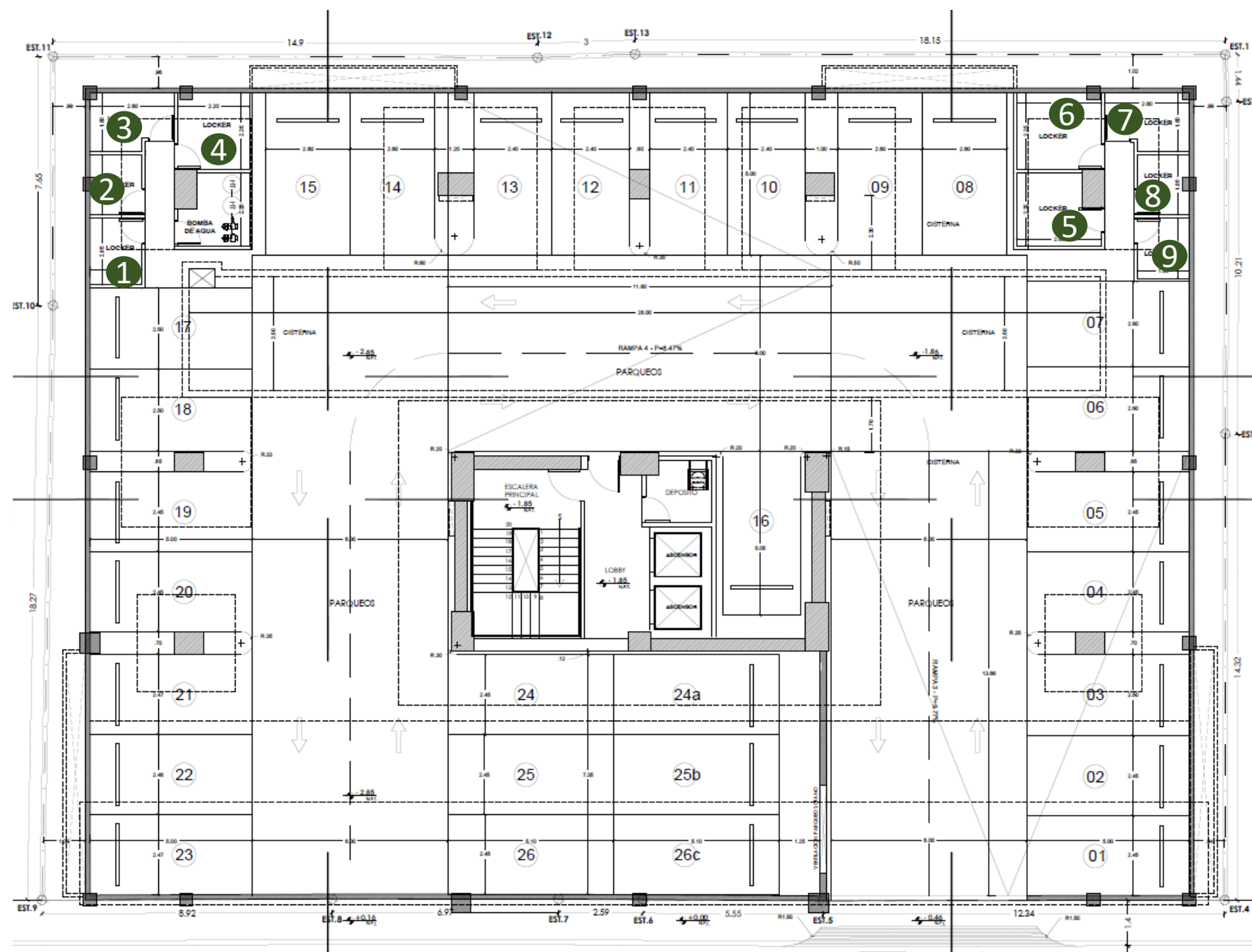
PLANTA ARQ. DE SOTANO
