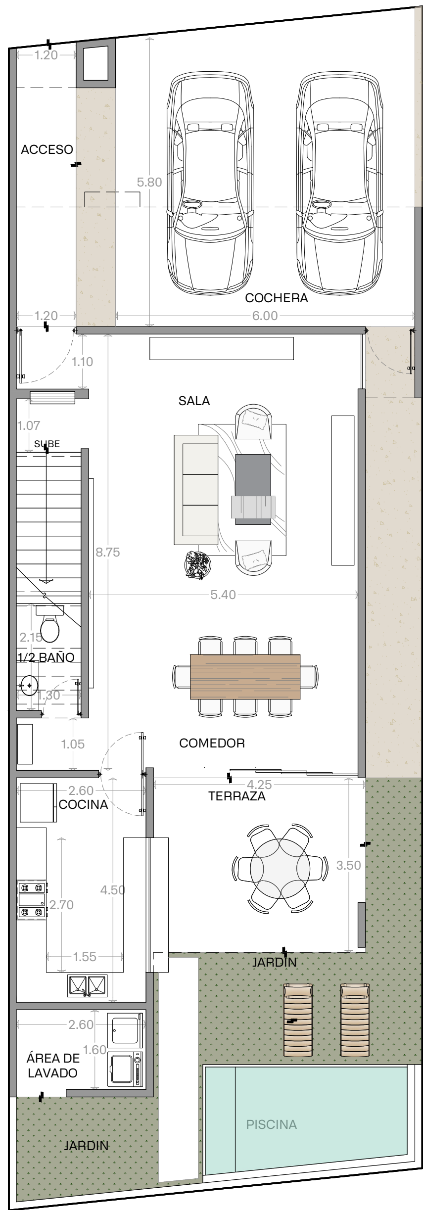
PLANTA BAJA
