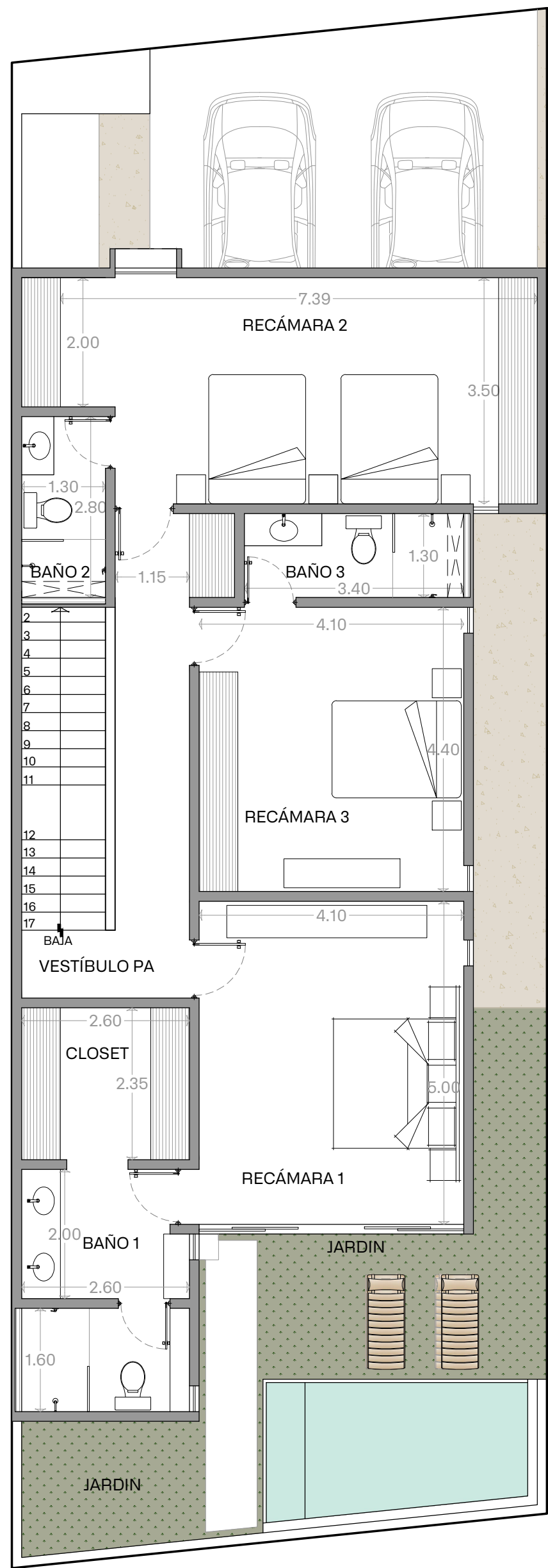
PLANTA ALTA
