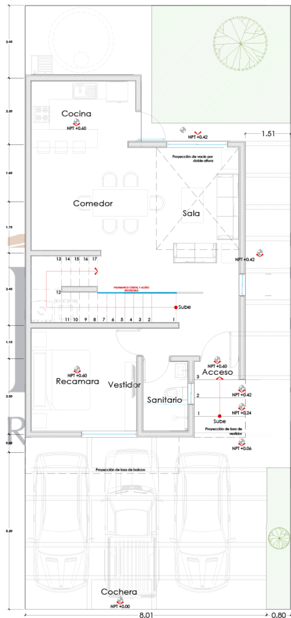
Arquitectónico Planta baja
