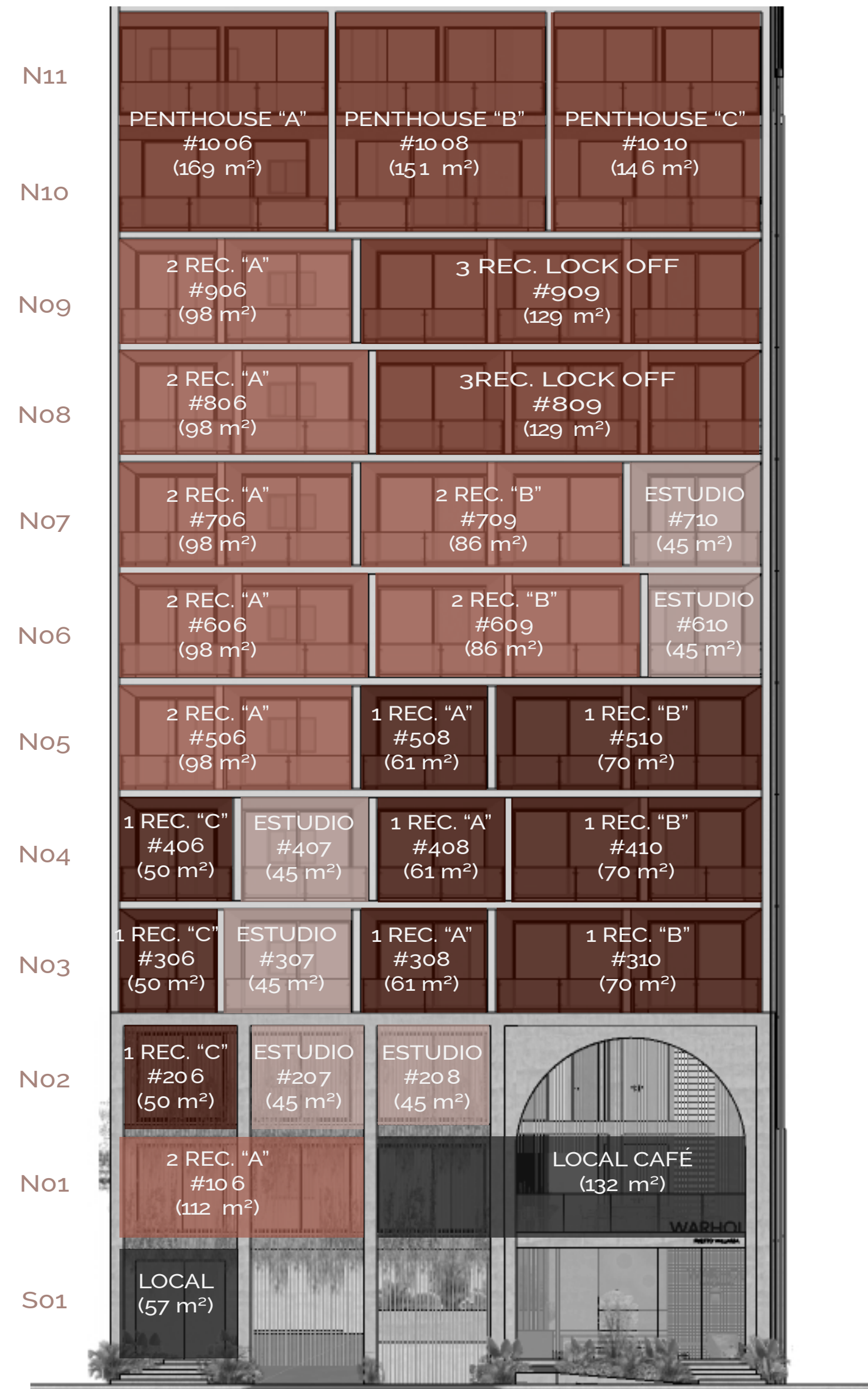
FACHADA FRONTAL
