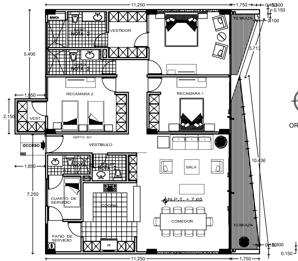
DEPARTAMENTO No.301, NIVEL 3+7.65
