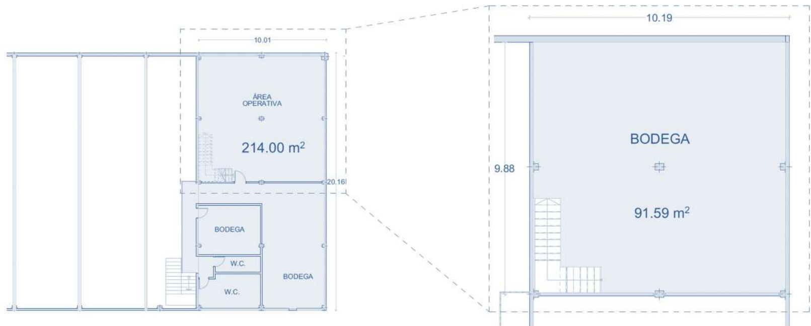
NIVEL 1
