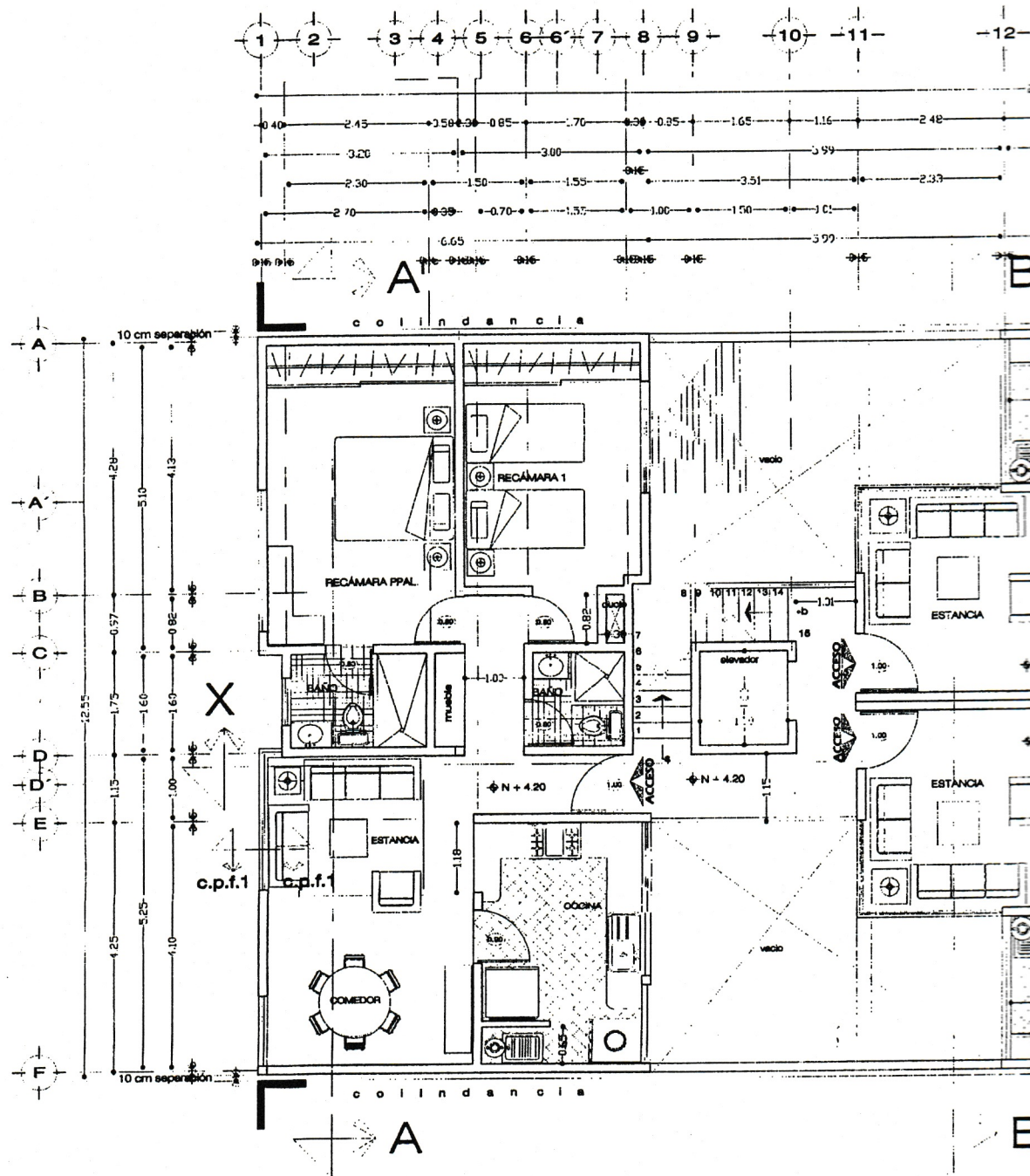
planta tipo
