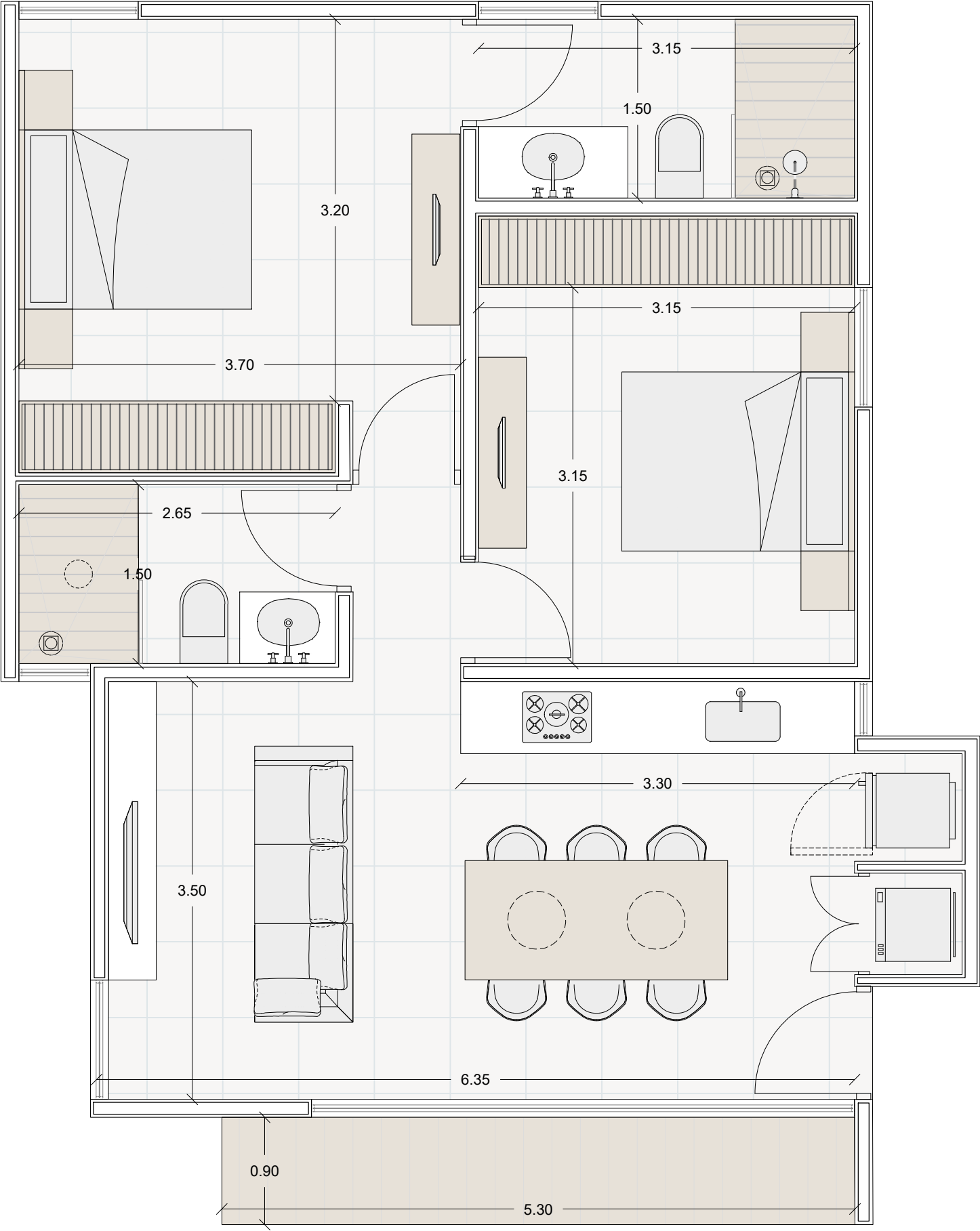
DEPARTAMENTO TIPO A
