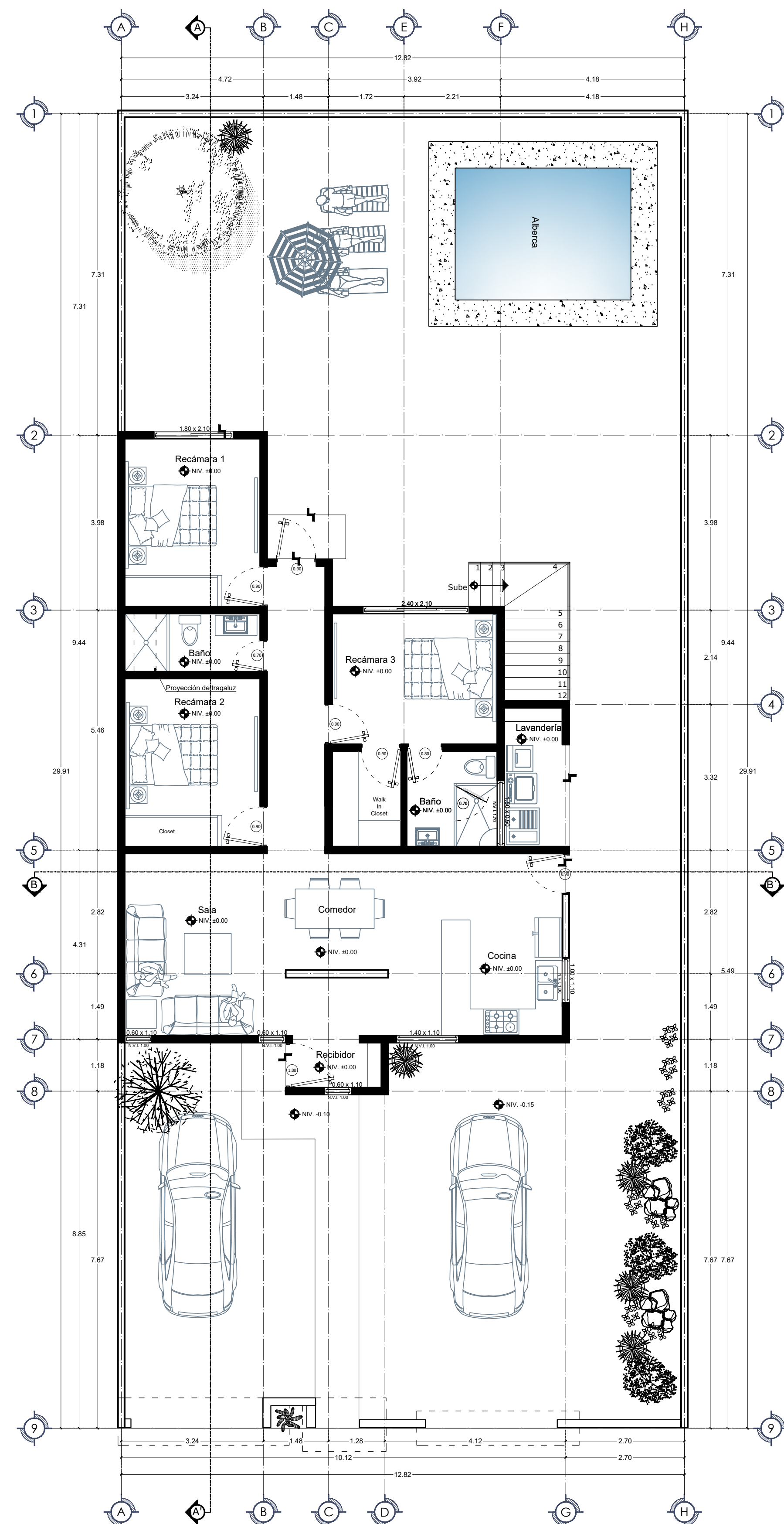
Planta Arquitectónica Baja Esc. 1:75 Área: 389.60 m 2
