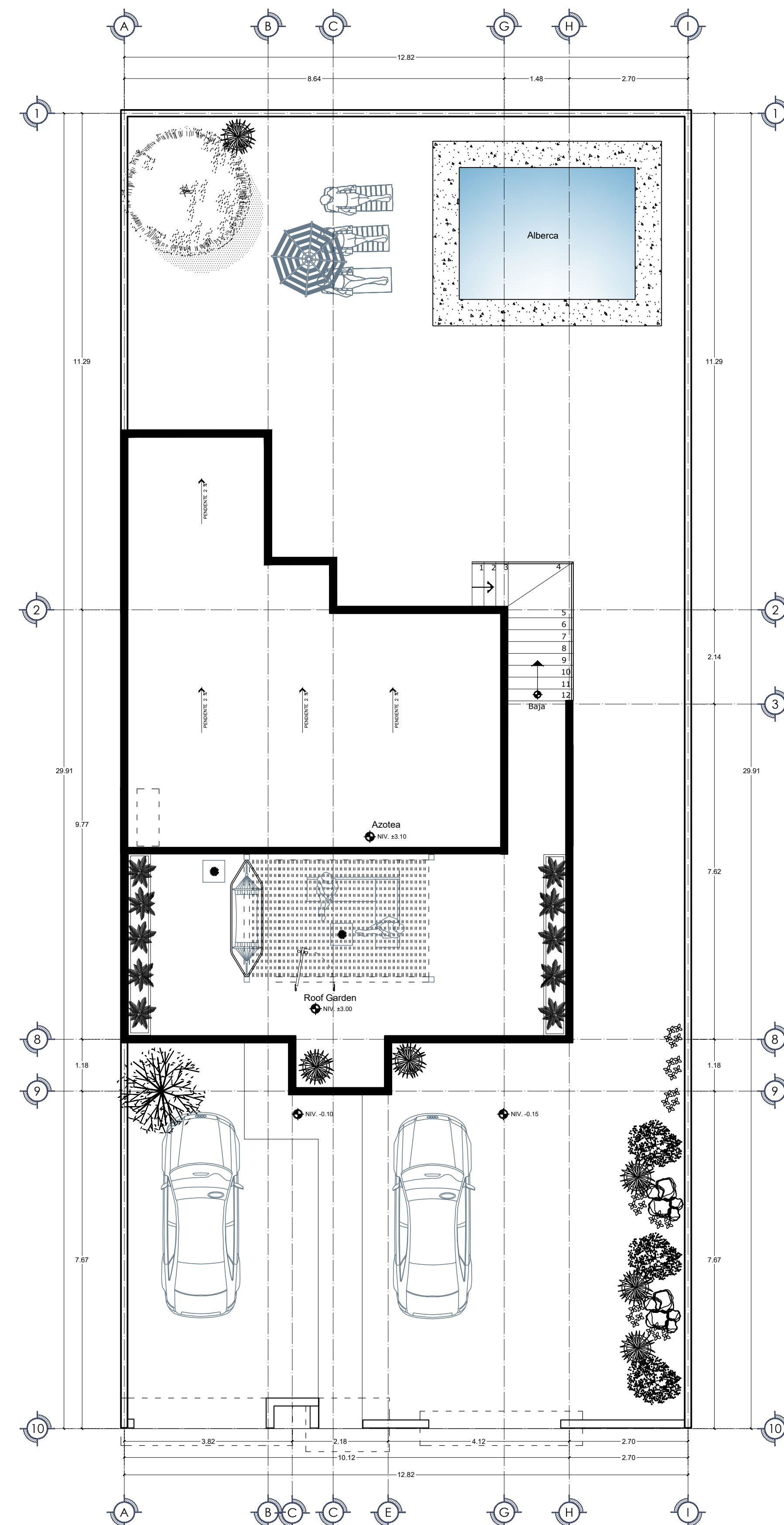
Planta Arquitectónica Alta Esc. 1:75 Área: 389.60 m 2
