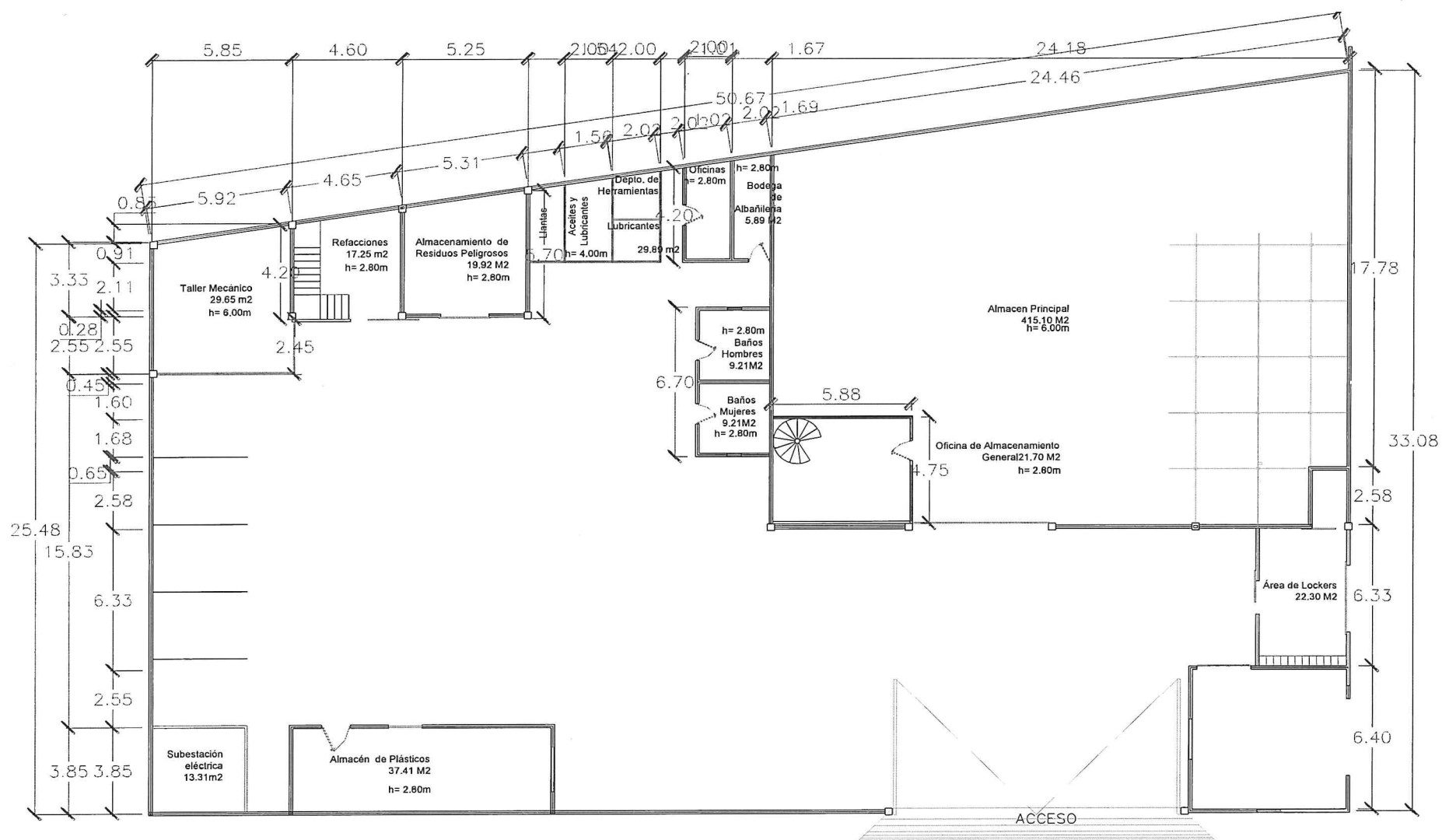
PLANTA BAJA ALMACEN PRINCIPAL Y TALLER DE MECANICA.
