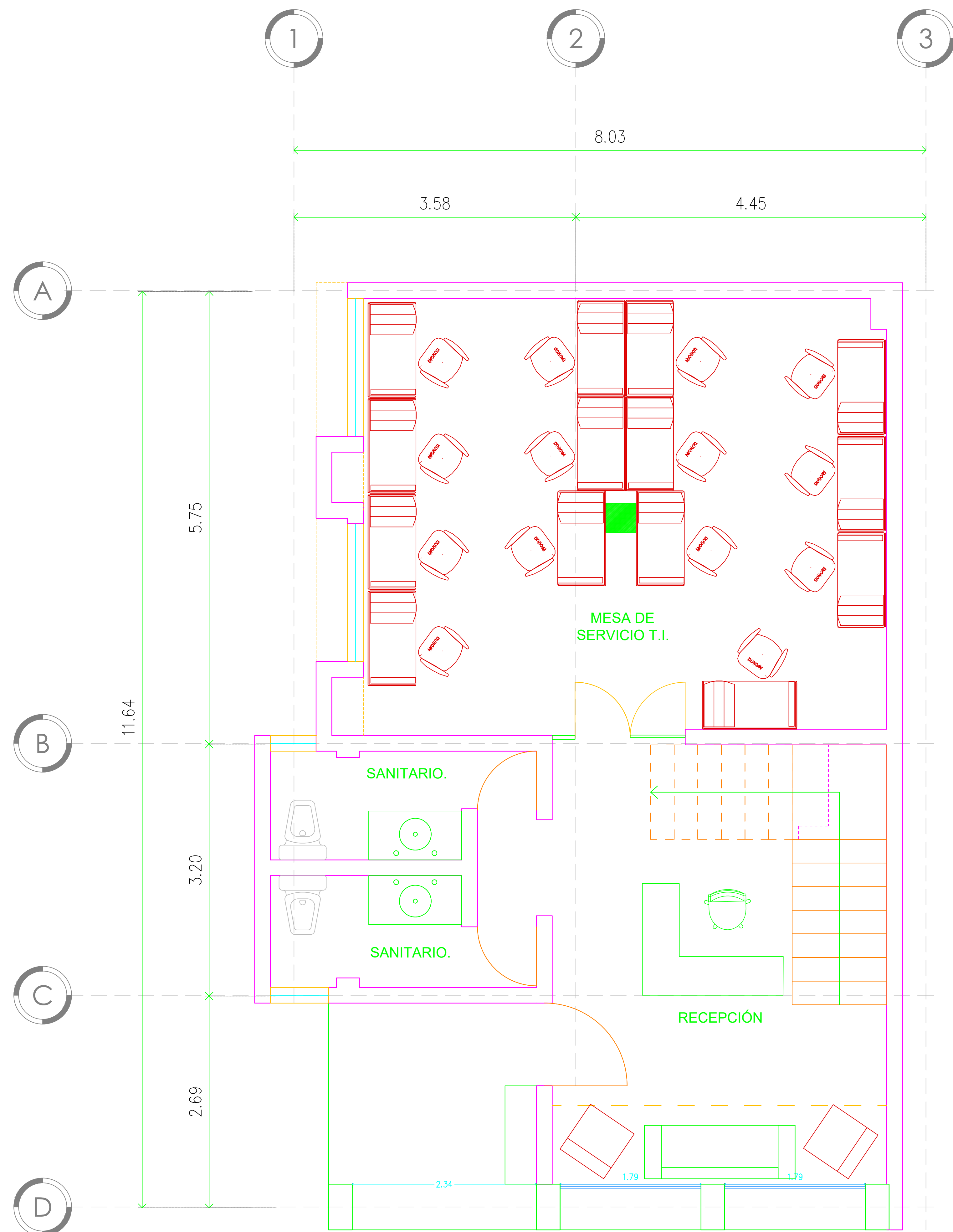
PLANTA BAJA
