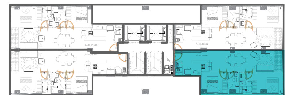
PLANTA ESQUEMÁTICA
