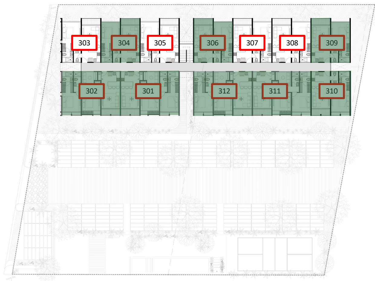
PLANTA ARQUITECTONICA – NIVEL 02
