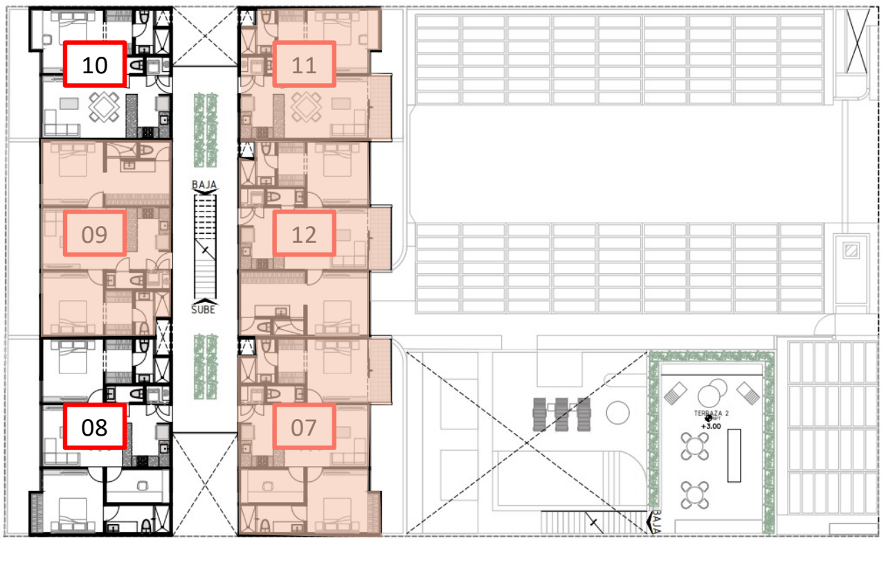
PLANTA ARQUITECTONICA – NIVEL 01
