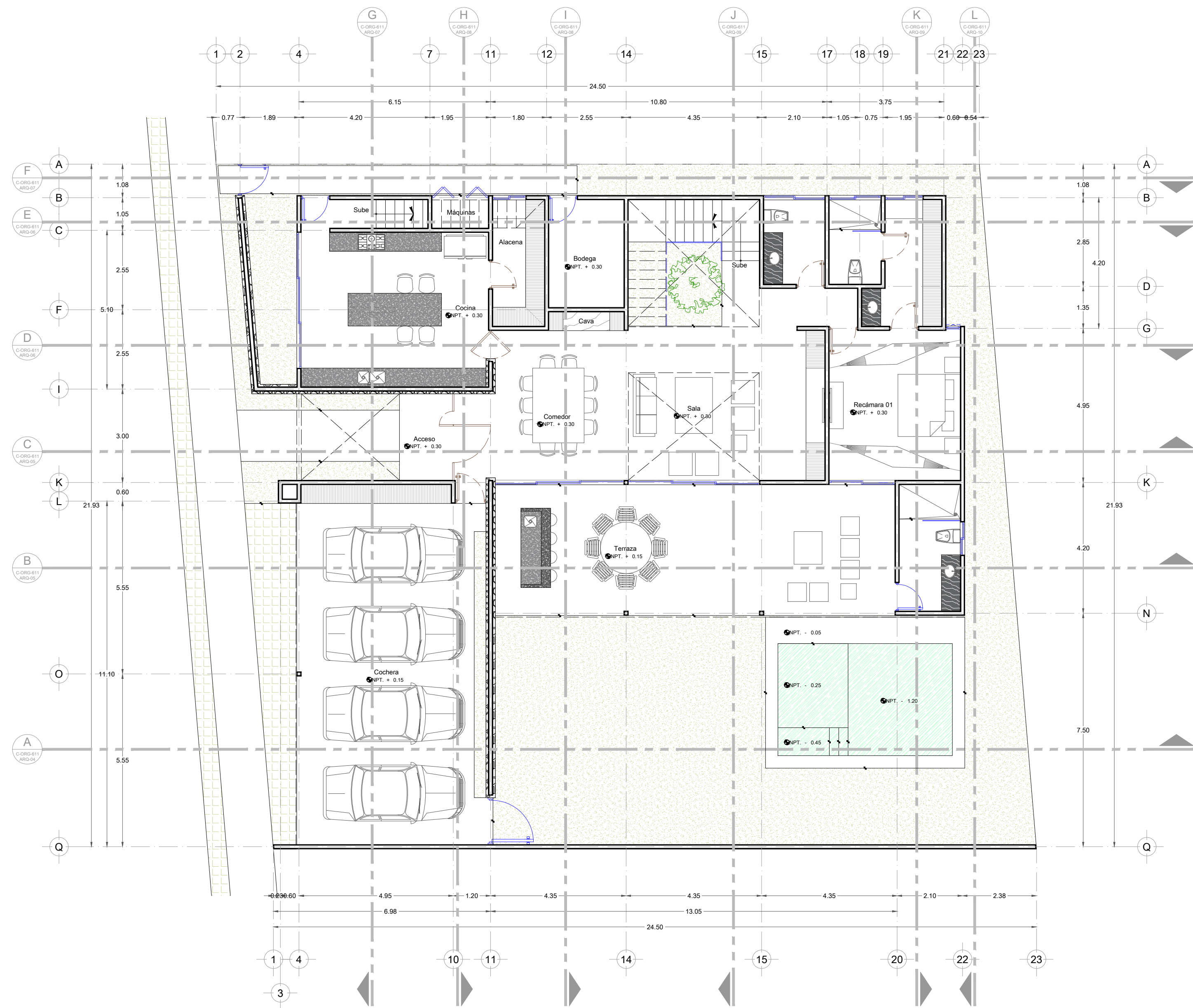
PLANTA BAJA
