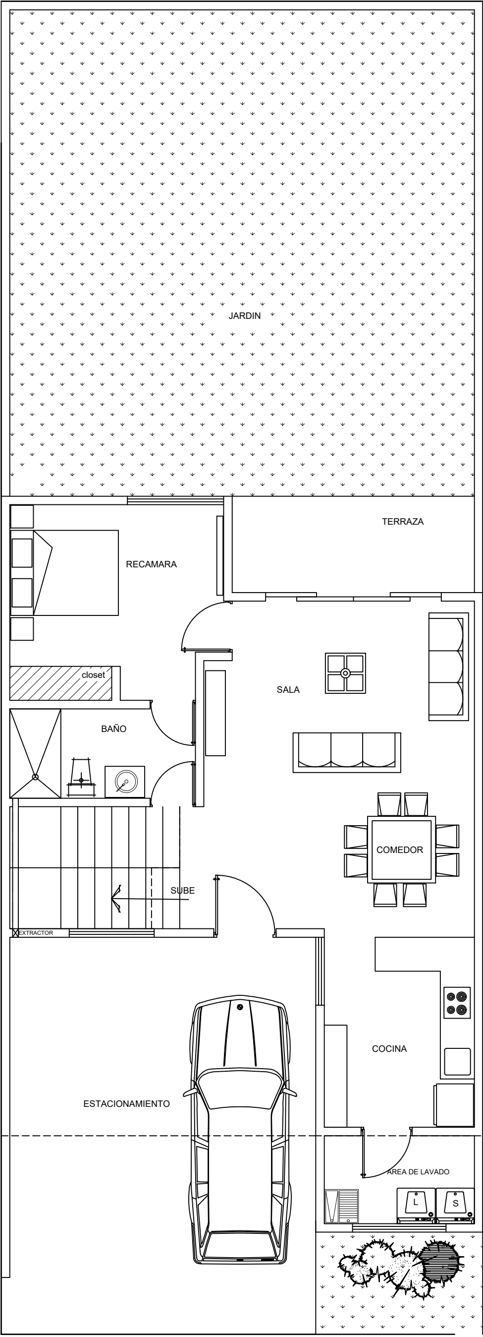
PLANTA BAJA
