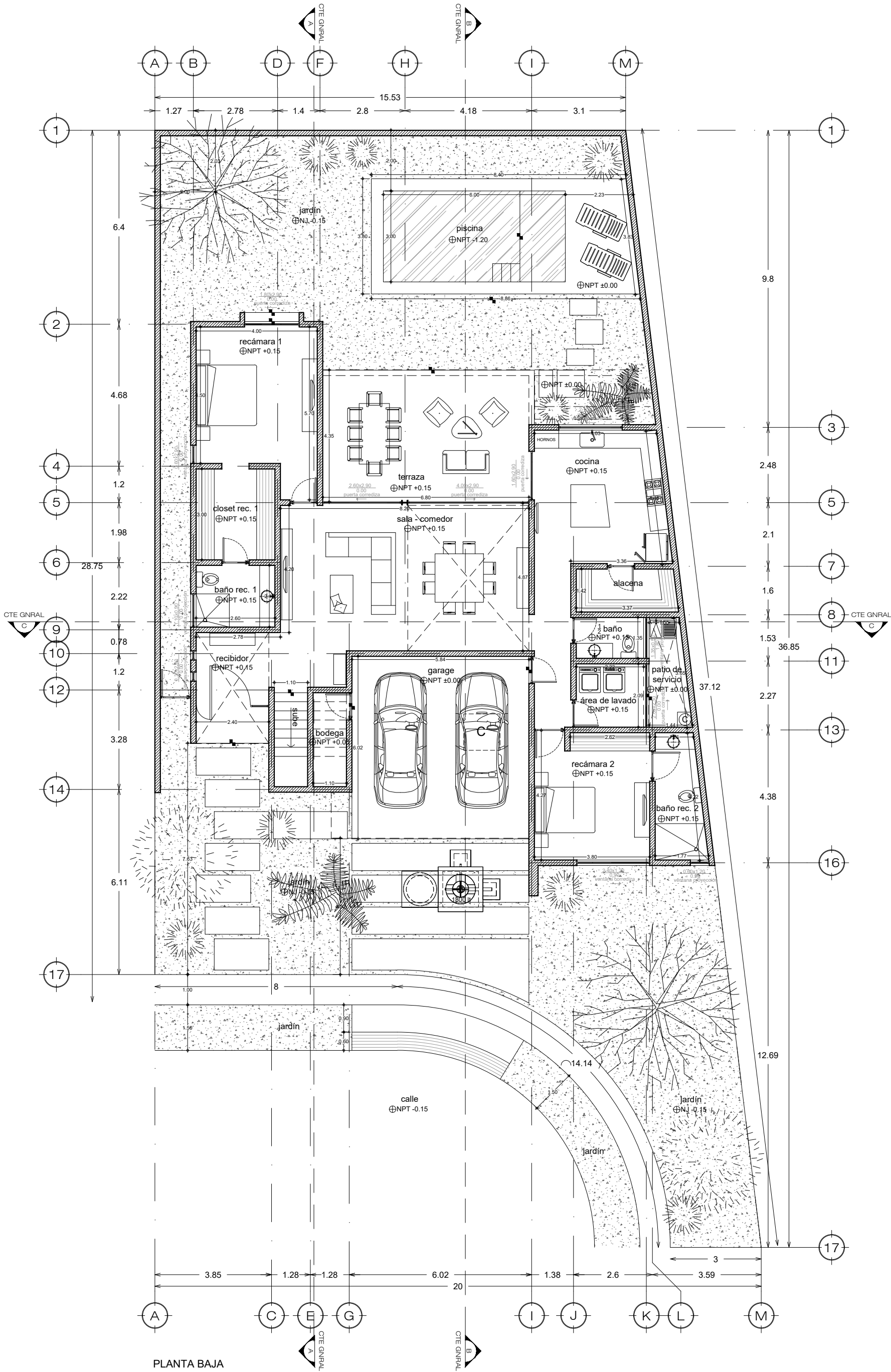
PLANTA BAJA área: 235.56m 2
