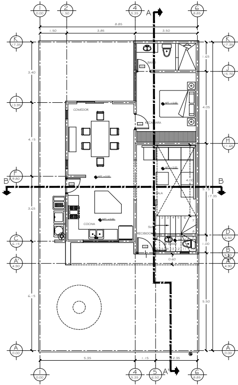
PLANTA BAJA 65.98 m2
