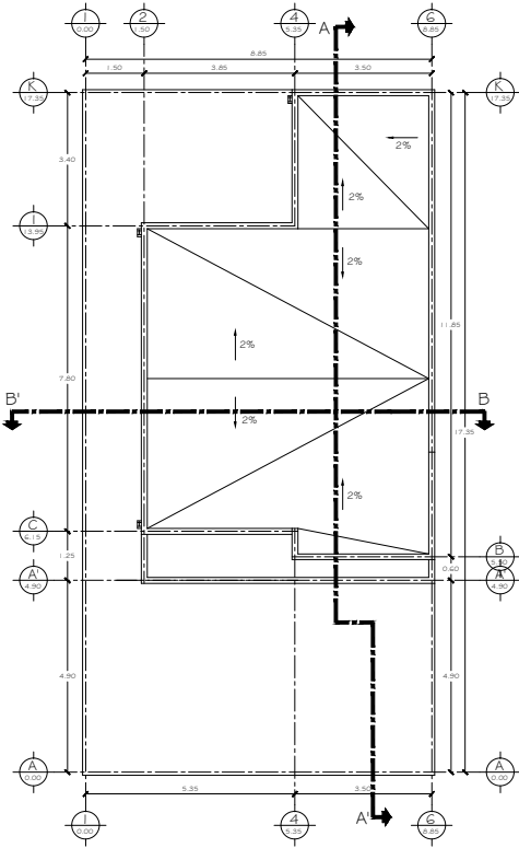
PLANTA DE AZOTEAS
