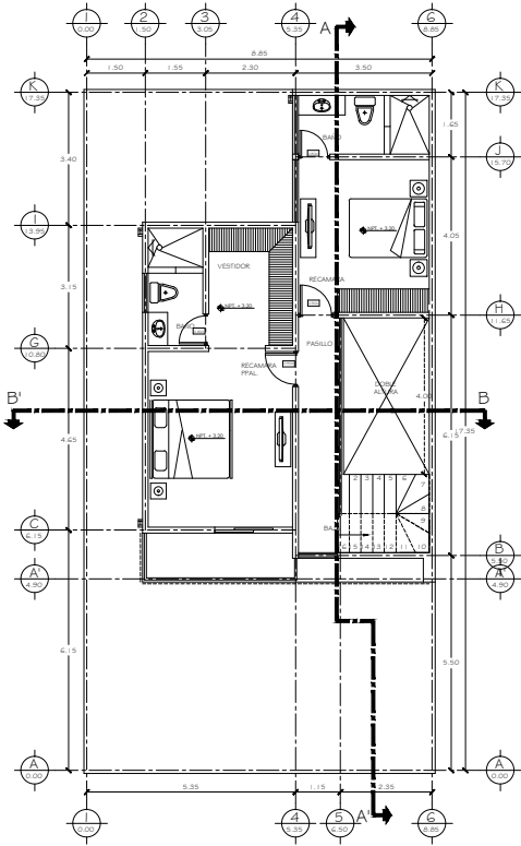
PLANTA ALTA 74.58 m2
