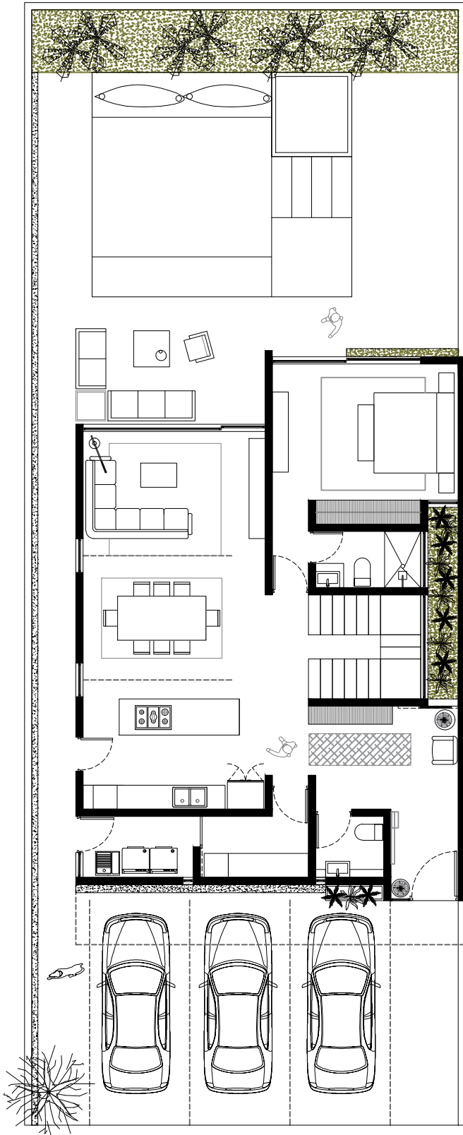
CASAS FIESTA MODELO 11X28 PLANTA BAJA
