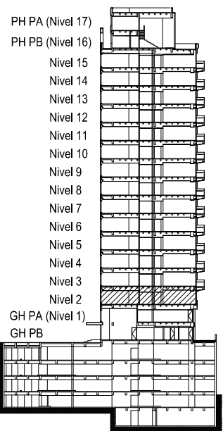
Corte esquemático s/e
