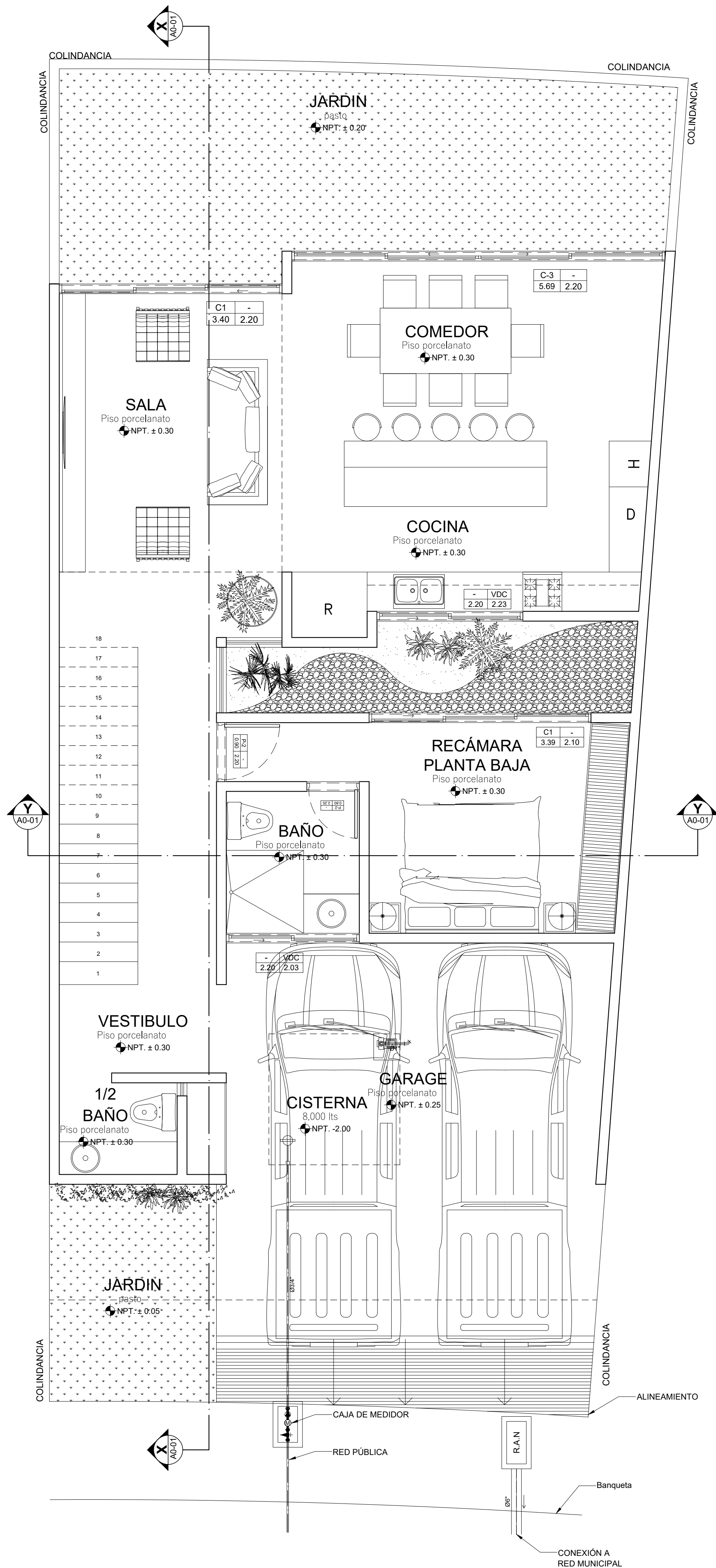
PLANTA BAJA ESC. 1:75
