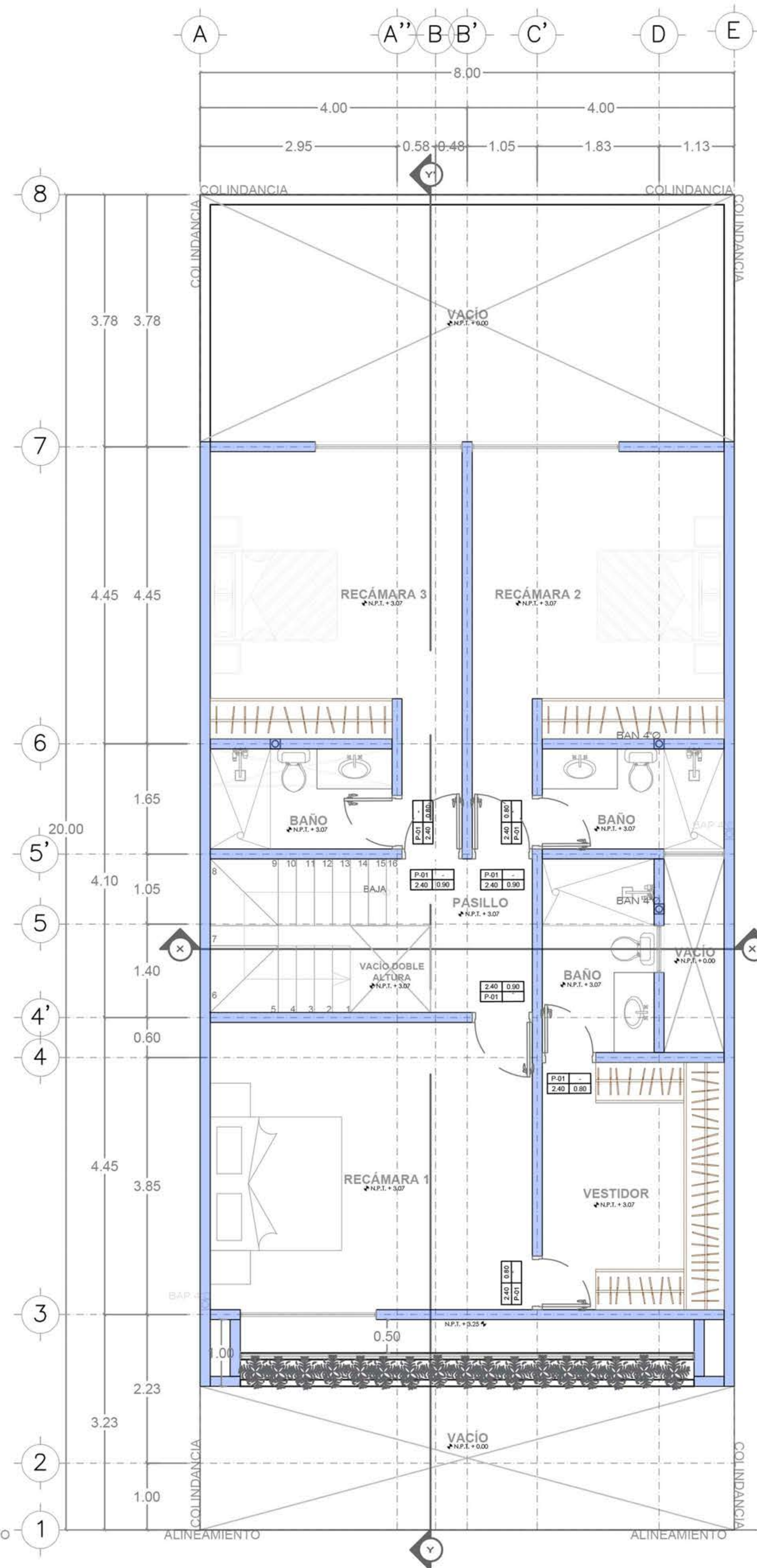
PLANTA ALTA
