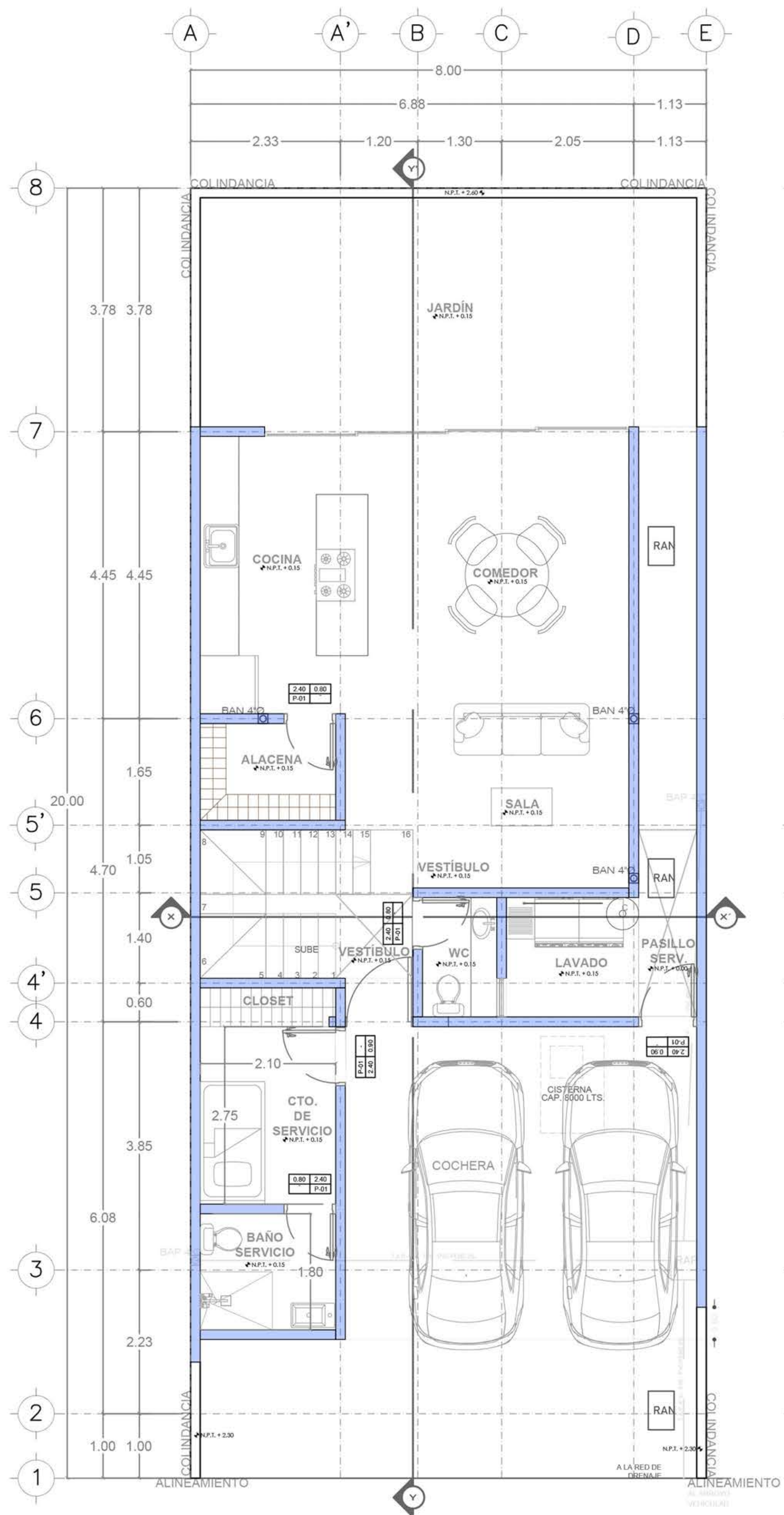
PLANTA BAJA
