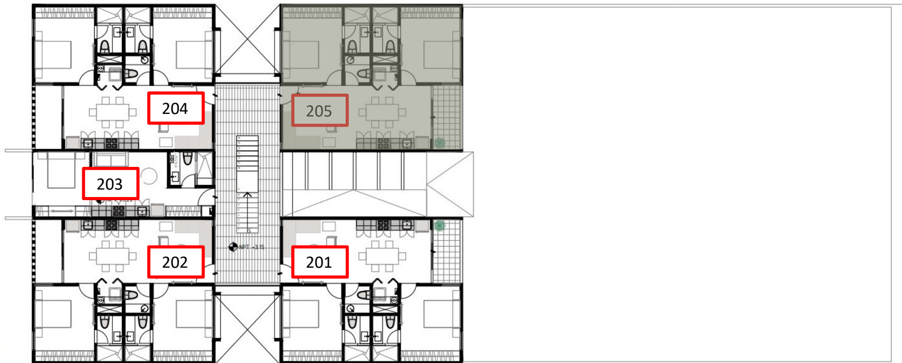
PLANTA ARQUITECTONICA – NIVEL 01
