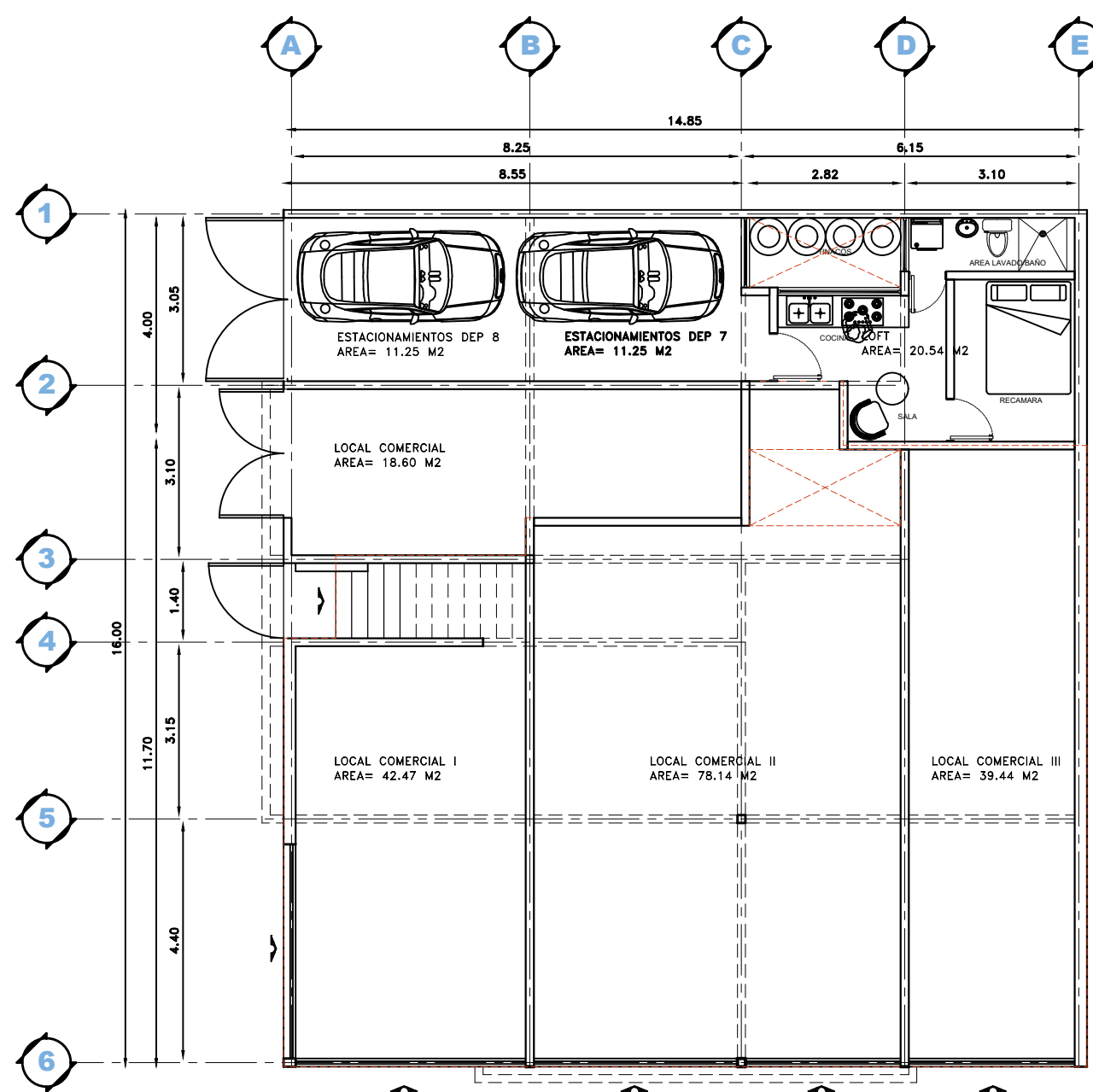
PLANTA BAJA
