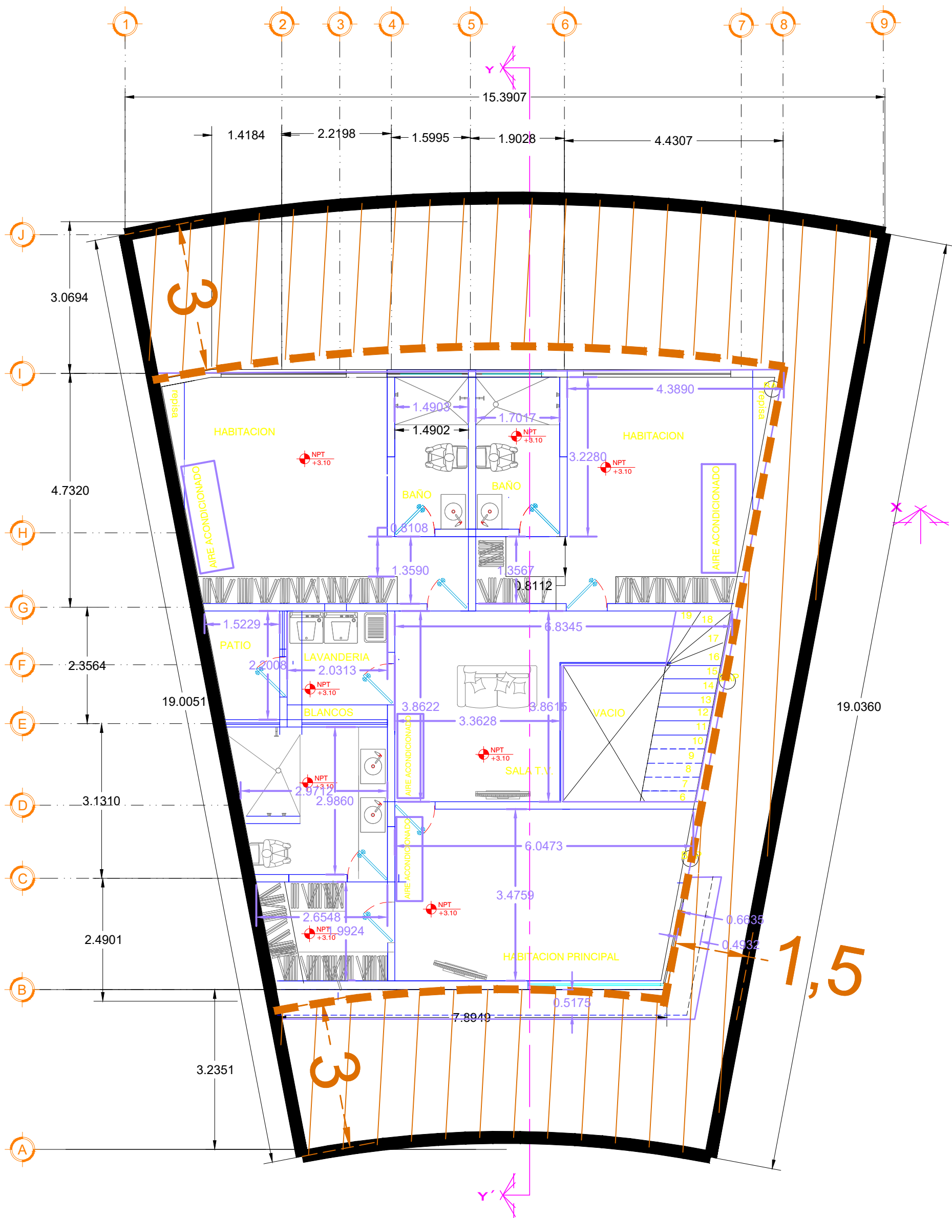
PLANTA BAJA
