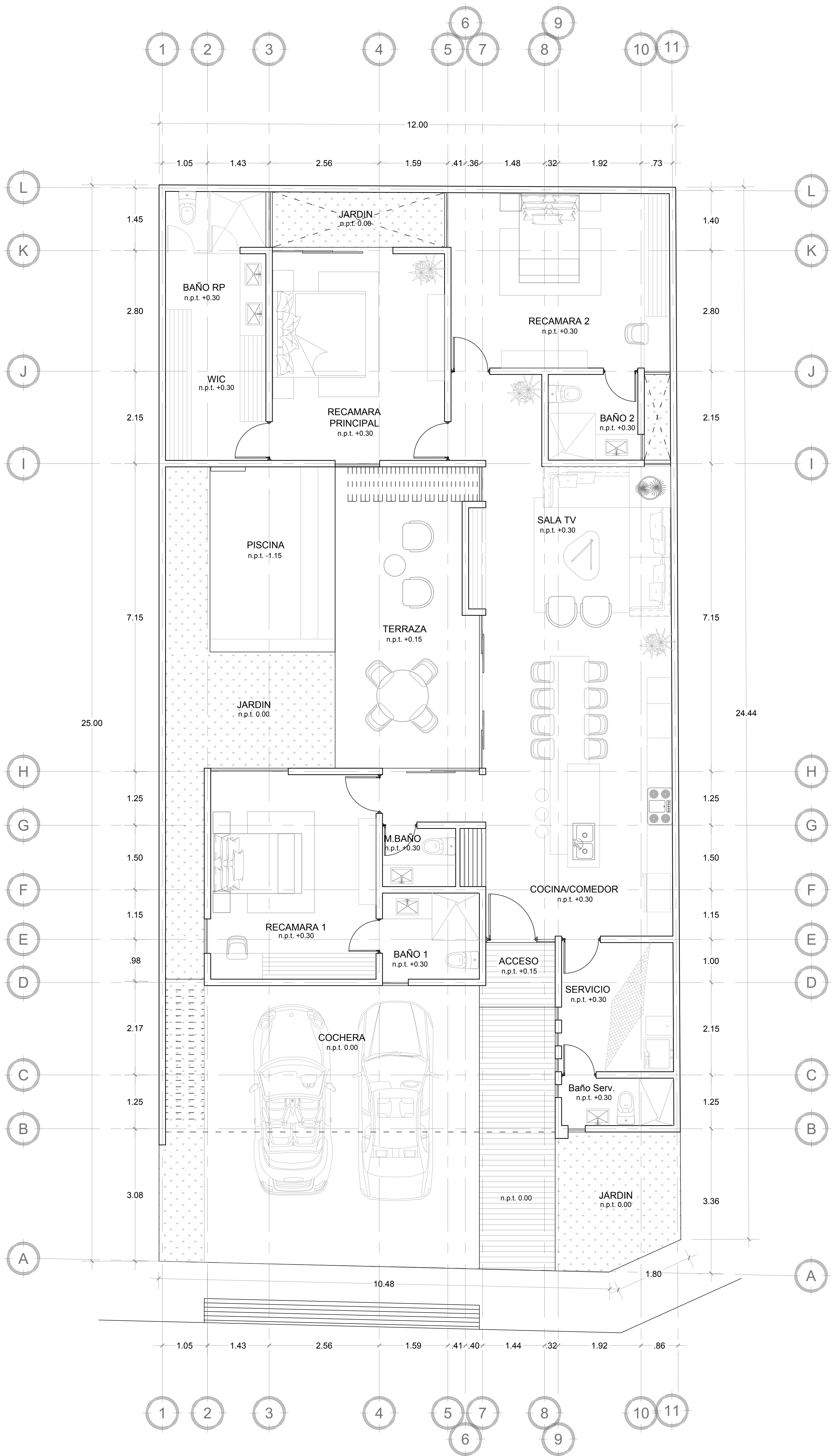
PLANTA ARQUITECTONICA
