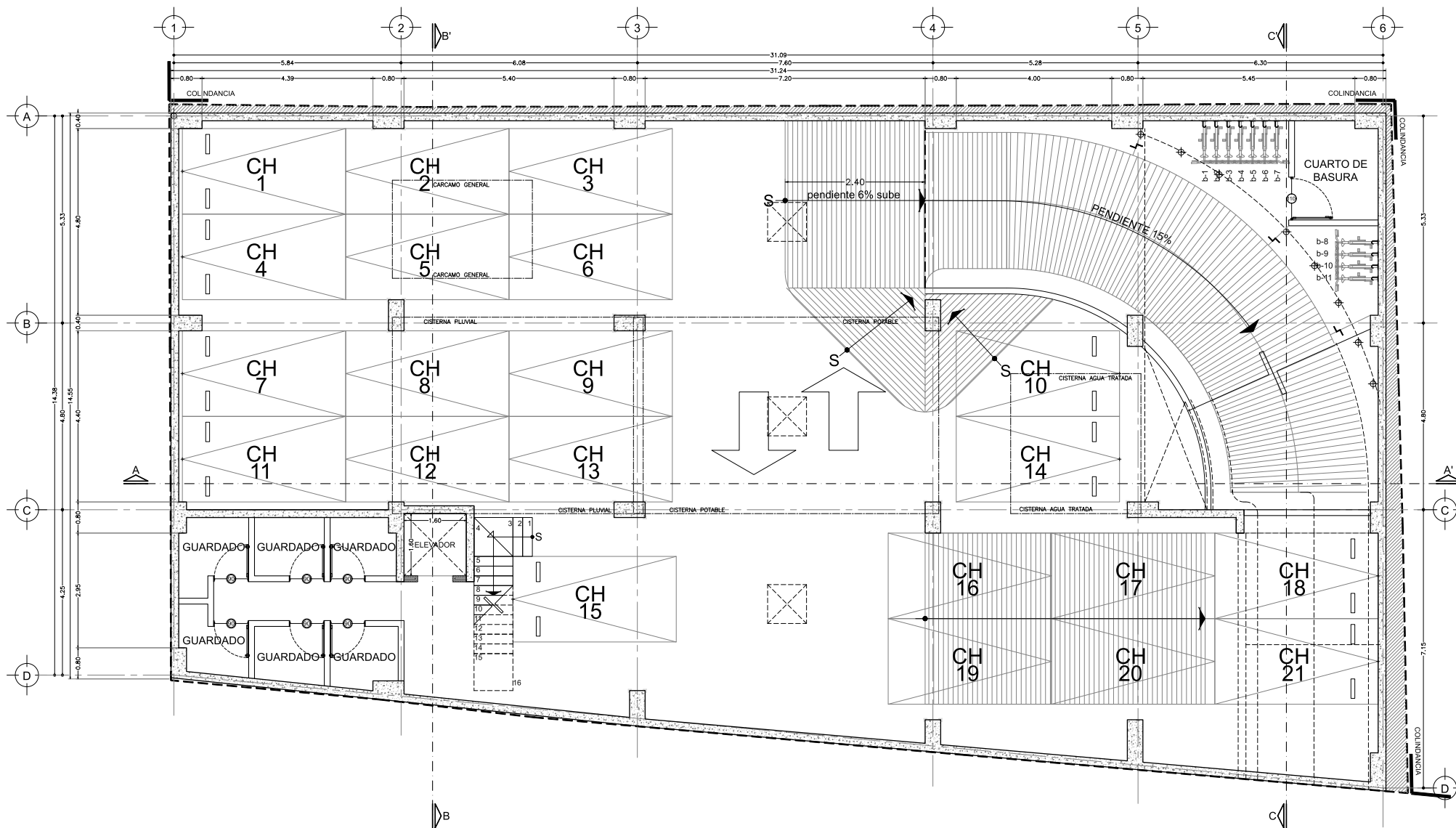
PLANTA SÓTANO N.P.T. -3.10
