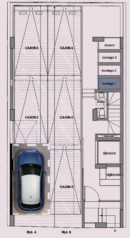
Nivel + 1
