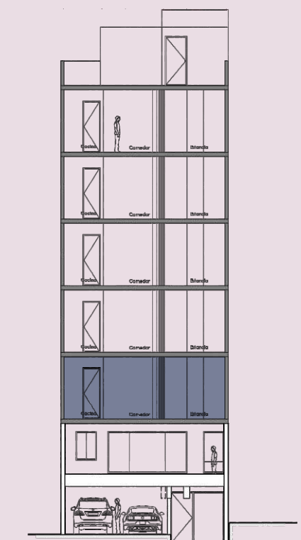
Nivel + 2
