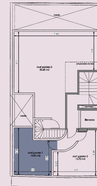
Planta azotea roof garden 1
