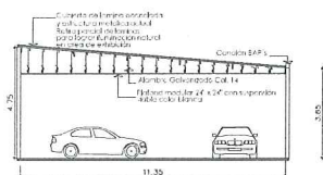
corte a-a (Dimensiones aproximadas) (3 MAYO 2012)
