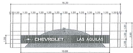
Marquesina Desplegada
