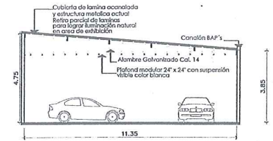
Corte Transversal
