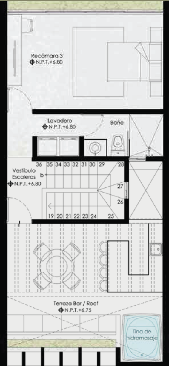
PLANTA ROOF
