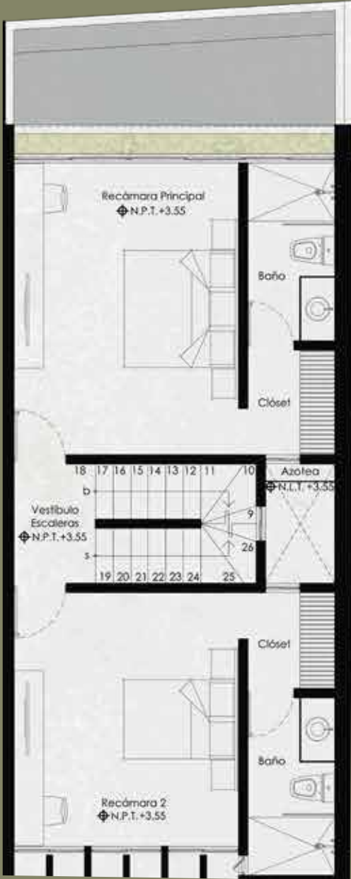
PRIMER NIVEL
