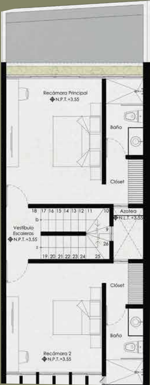
PRIMER NIVEL
