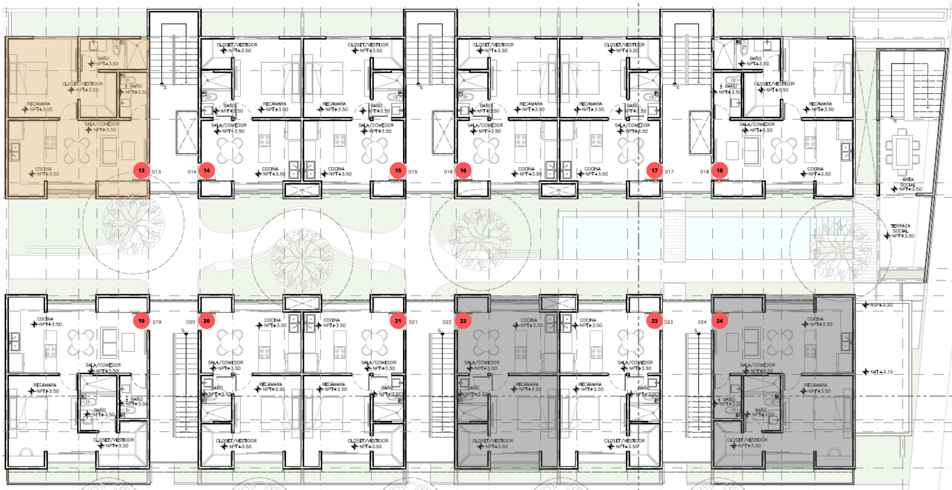
PLANTA NIVEL 1
