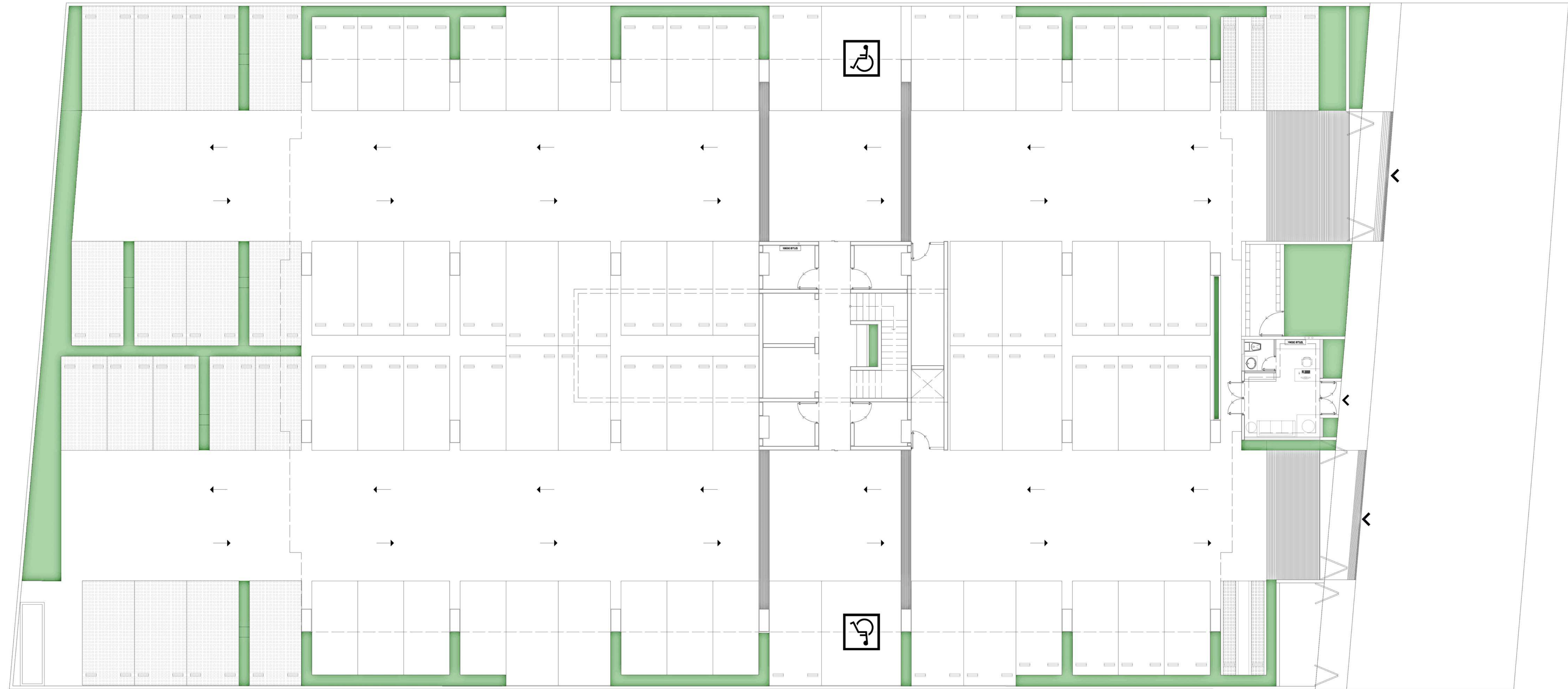
PLANTA ESTACIONAMIENTO
