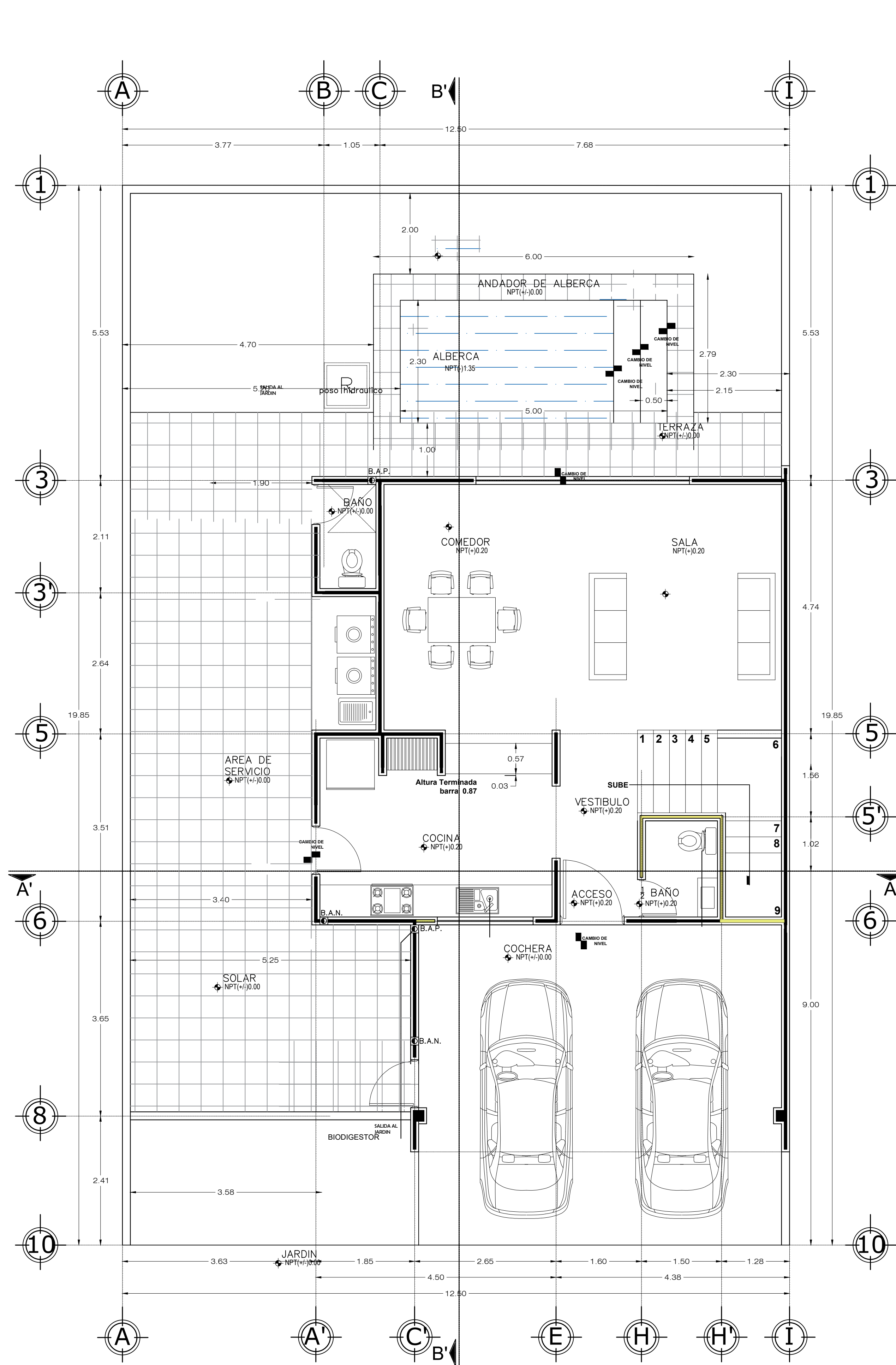
Planta Baja Proyecto Arquitectónico ESC. 1:100
