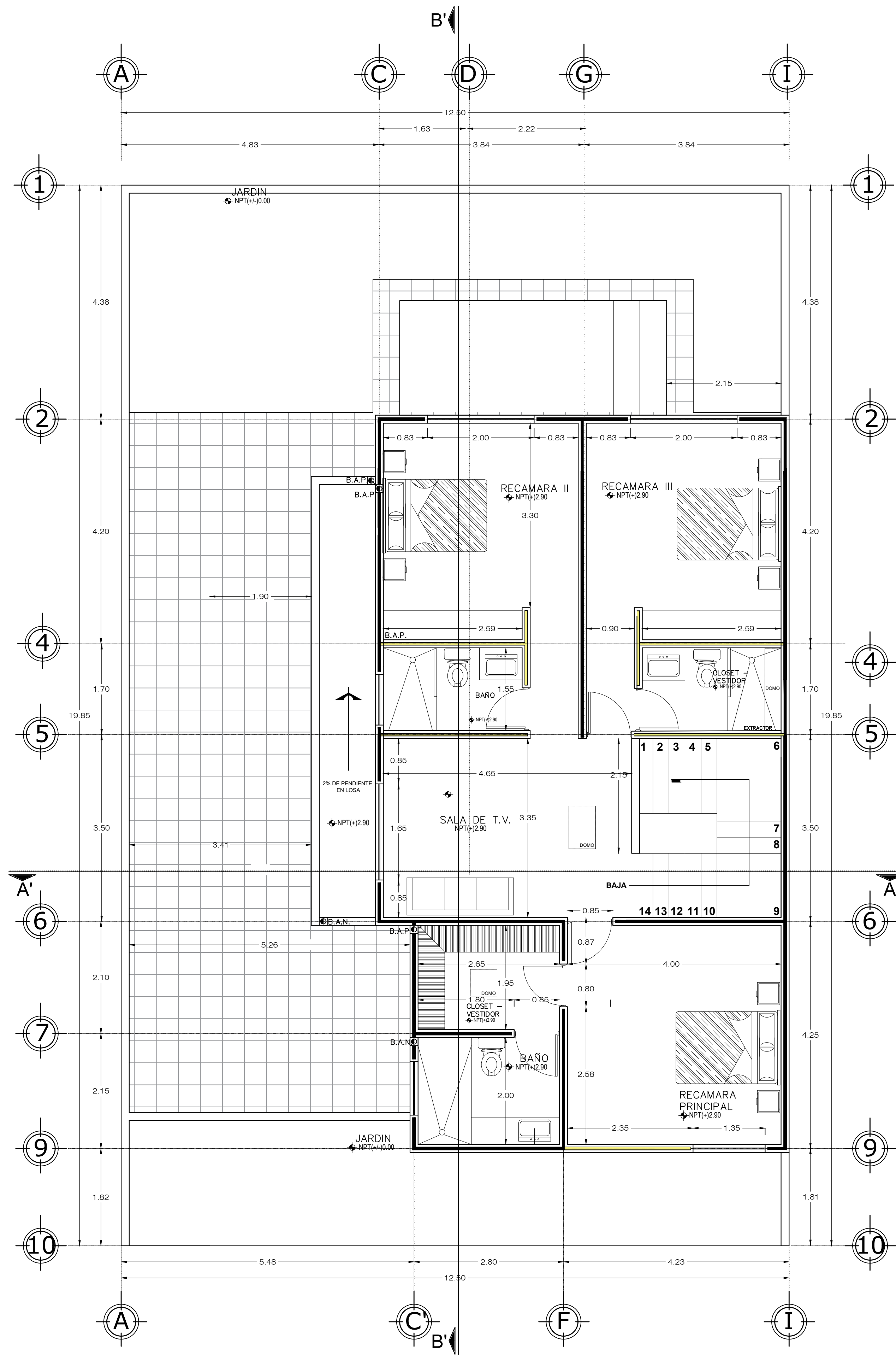
Planta Alta Proyecto Arquitectónico ESC. 1:100
