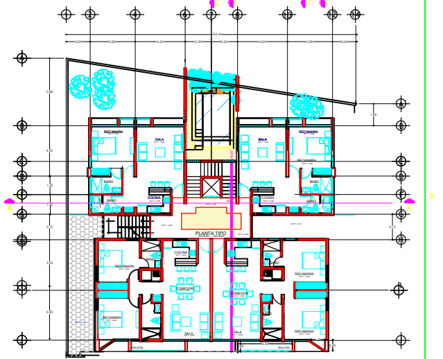
CUARTO NIVEL (NIVEL +12.90) 350.00 M2 2 departamentos Tipo 1. 64.90m2 2 departamentos Tipo 2. 84.70m2
