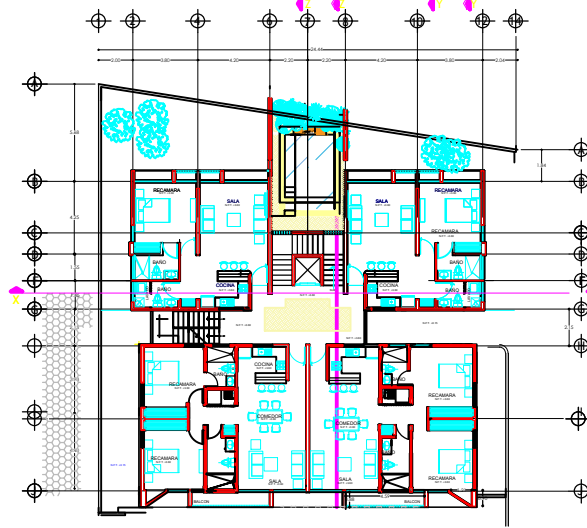
TERCER NIVEL (NIVEL +9.80) 350.00 M2 2 departamentos Tipo 1. 64.90m2 2 departamentos Tipo 2. 84.70m2
