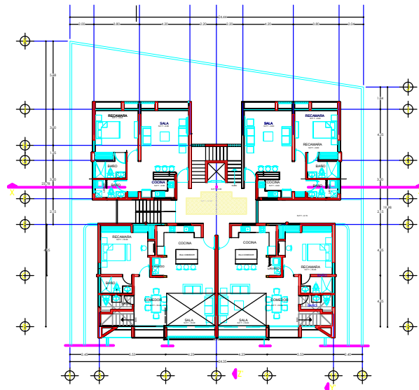
QUINTO NIVEL (NIVEL +16.00) 350.00 M2 2 departamentos Tipo 1. 64.90m2
