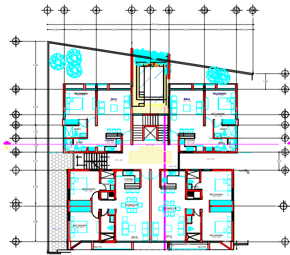
SEGUNDO NIVEL (NIVEL +6.70) 350.00 M2 2 departamentos Tipo 1. 64.90m2 2 departamentos Tipo 2. 84.70m2
