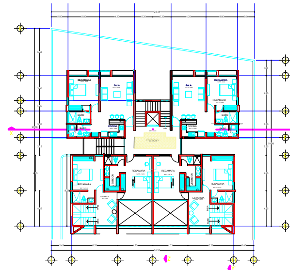
SEXTO NIVEL (NIVEL +19.10) 350.00 M2 2 departamentos Tipo 1. 64.90m2
