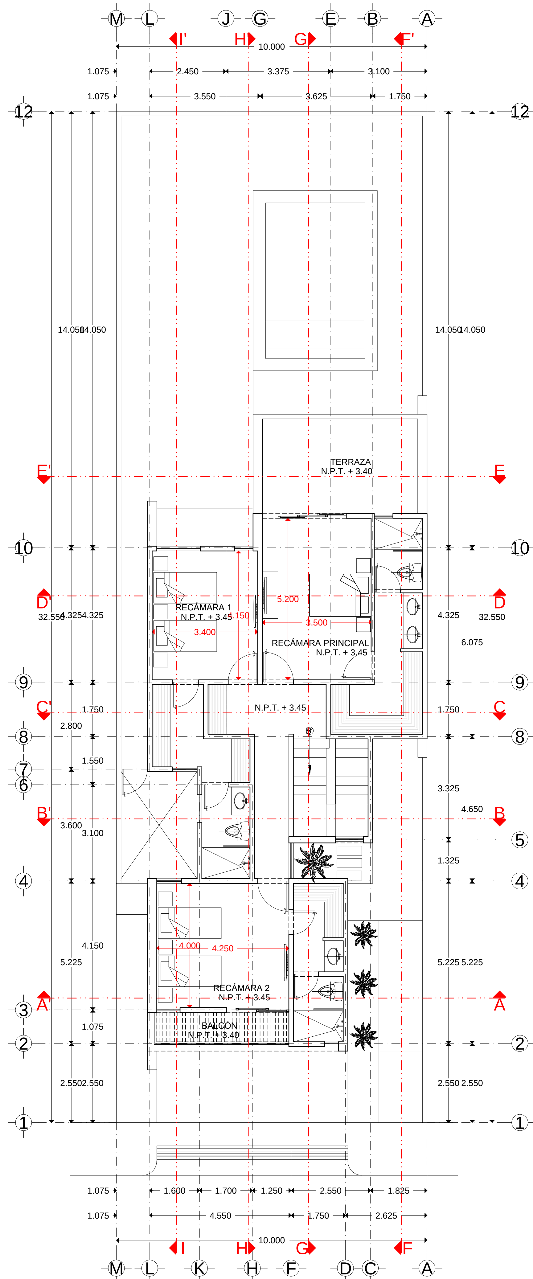
PLANTA PRIMER NIVEL. 121.50 M 2
