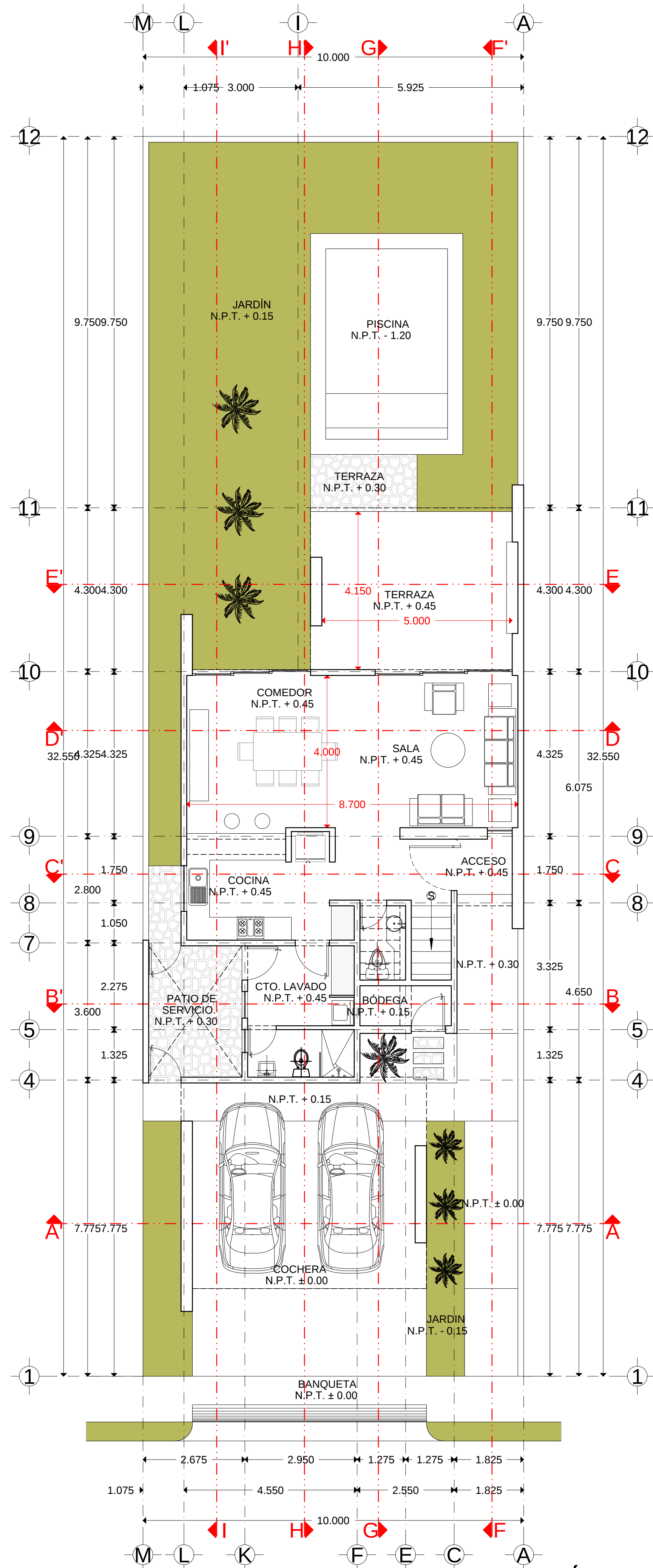
PLANTA ARQUITECTÓNICA. 137.50 M 2
