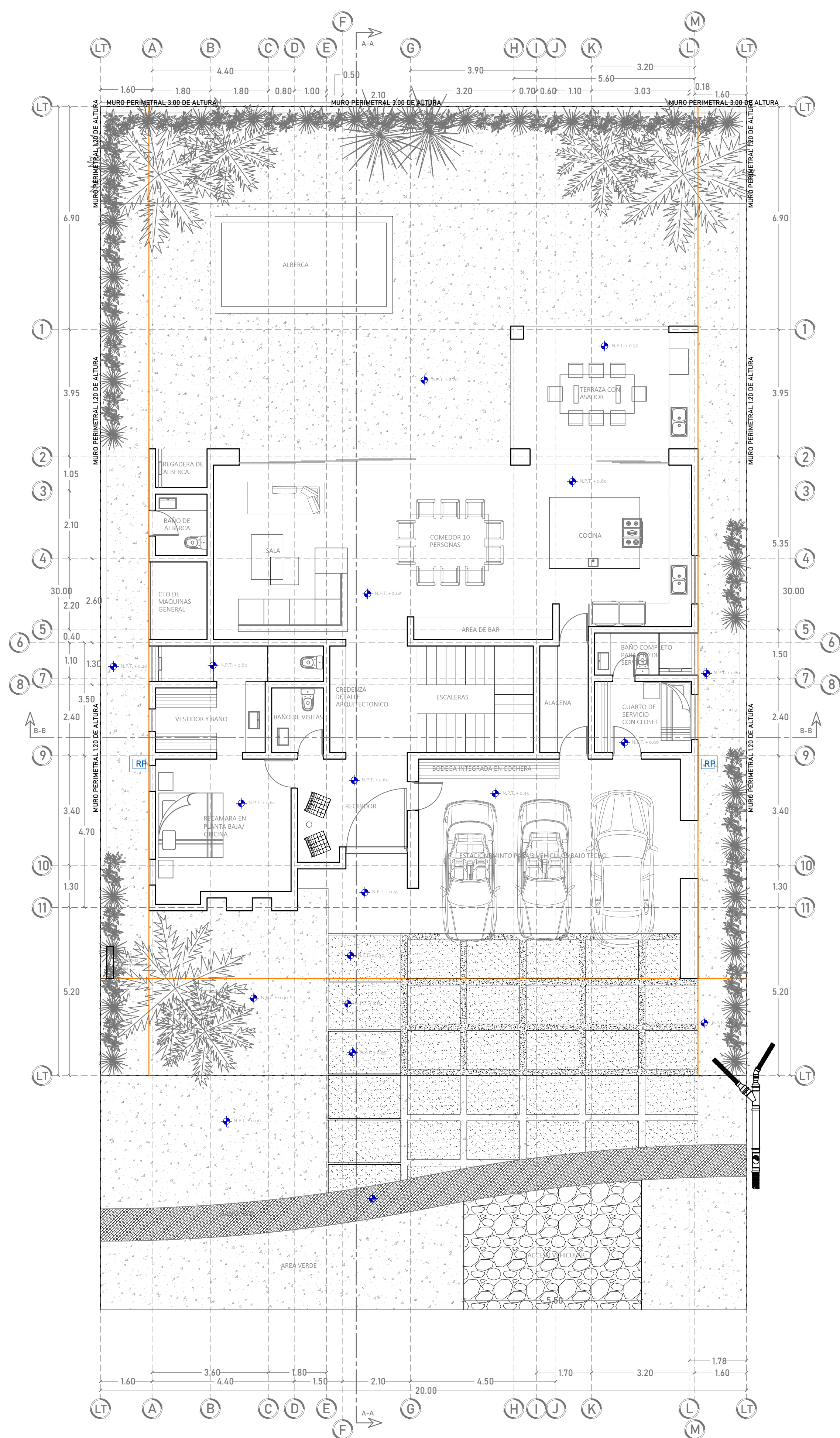
CUTZAM YVR 11 L42 ARQUITECTONICO NIVEL 1
