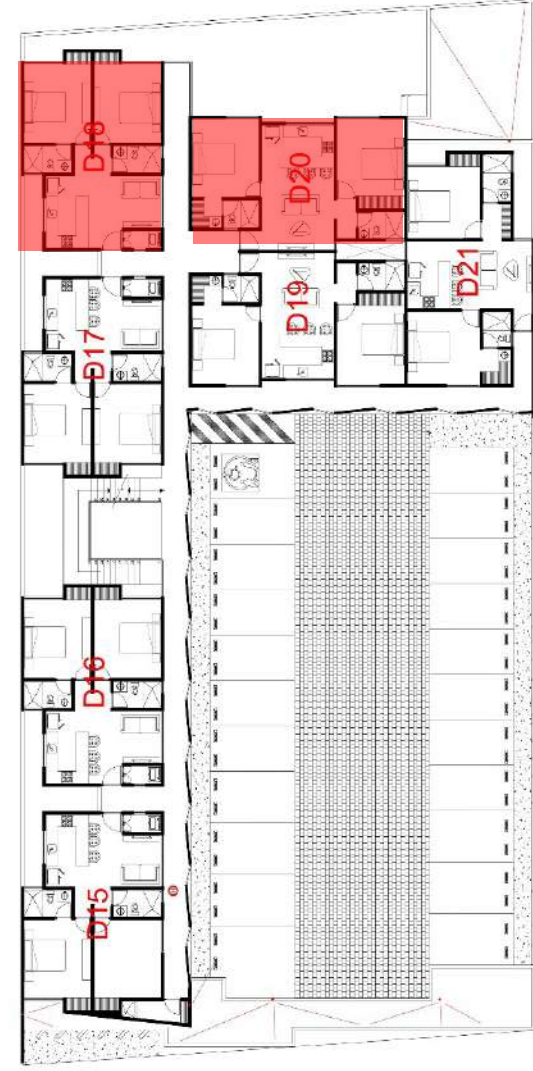
PLANTA SEGUNDO NIVEL
